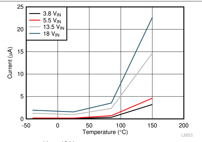
图 7-6. Shutdown Current
