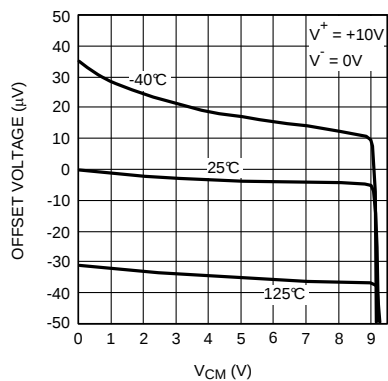
图 3. 失调电压与 V_{\text{CM}} 间的关系
