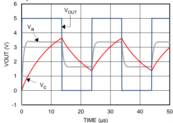
图 25. 方波振荡器输出波形
