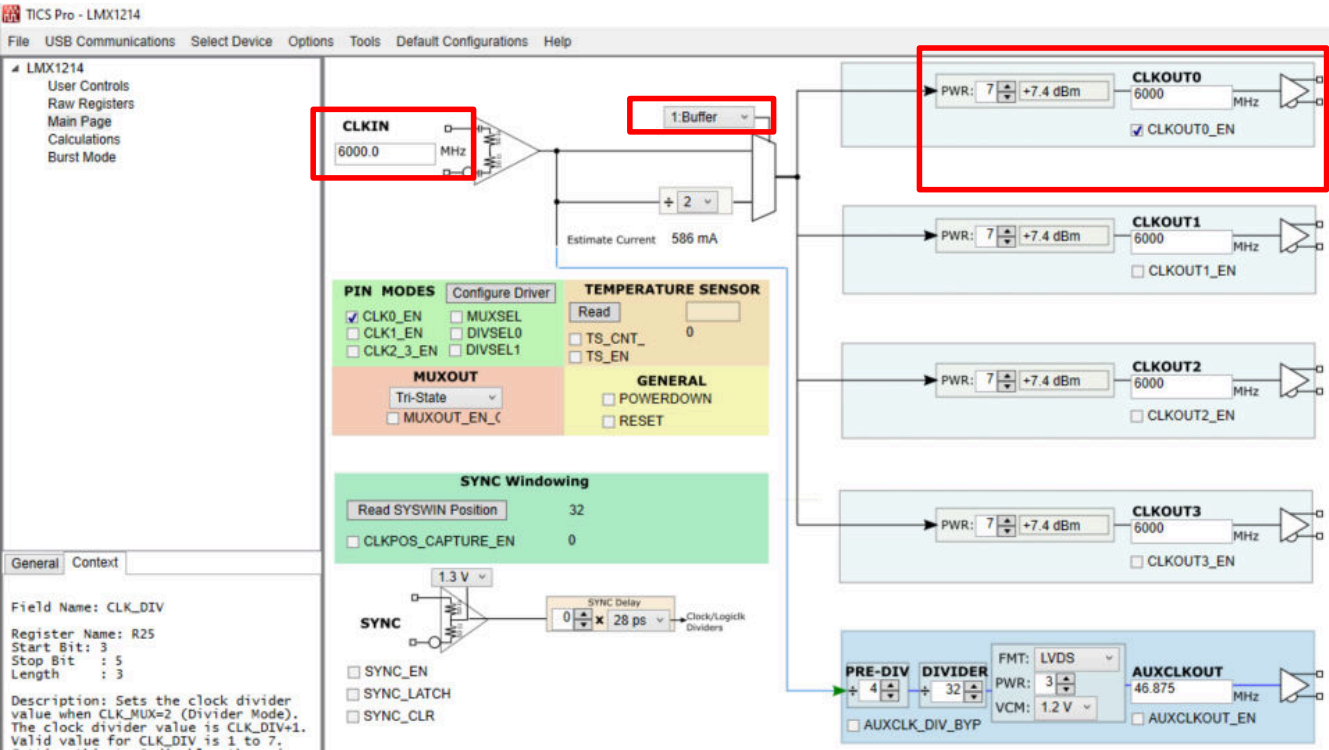
图 8-7. LMX1214 TICS Pro 设置
