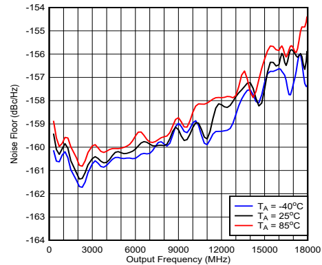
图 5-5. 缓冲器模式下的本底噪声
