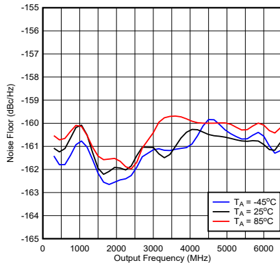
图 5-6. 分频器模式下的本底噪声
