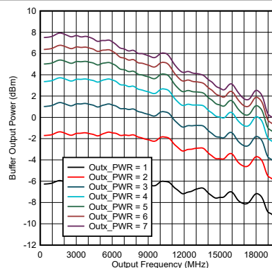
图 5-9. 缓冲器模式单端输出功率与功率代码间的关系
