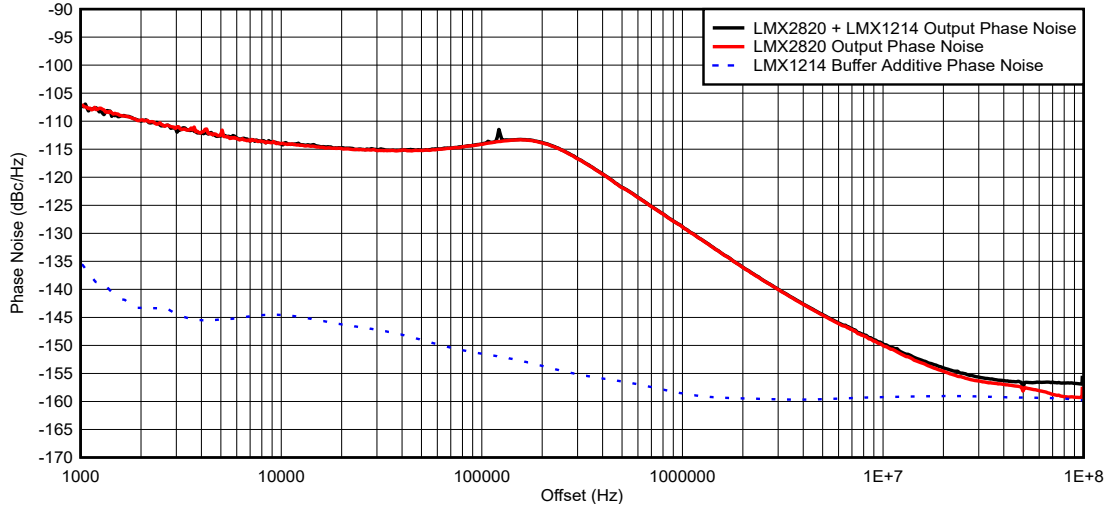
图 8-8. LMX1214 缓冲器输出
