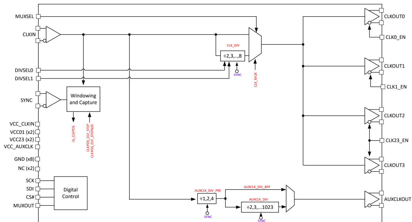
图 6-1. 功能方框图
