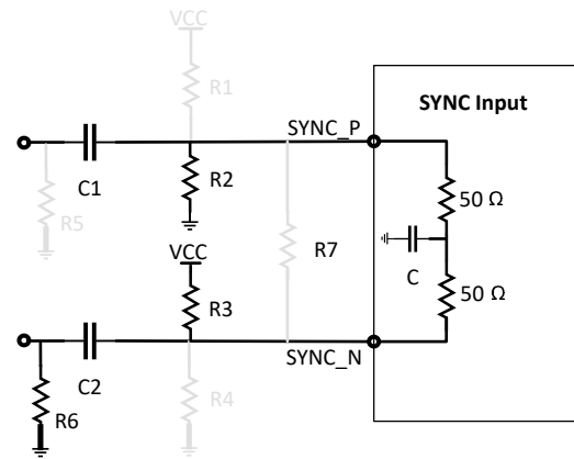
图 8-3. 交流耦合单端输入
