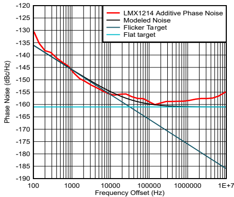
图 5-4. 6GHz 时的 LMX1214 闪烁噪声
