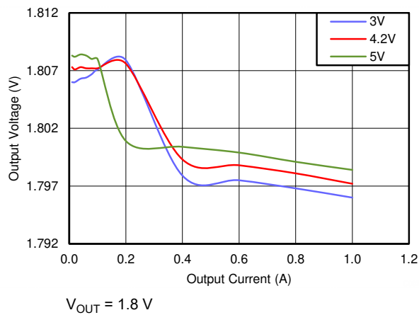
图 8-7. Regulation, AUTO Mode
