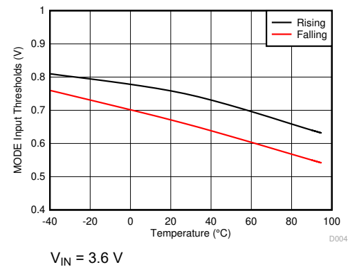
图 6-4. MODE Input Thresholds
