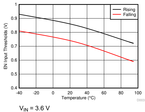
图 6-3. EN Input Thresholds
