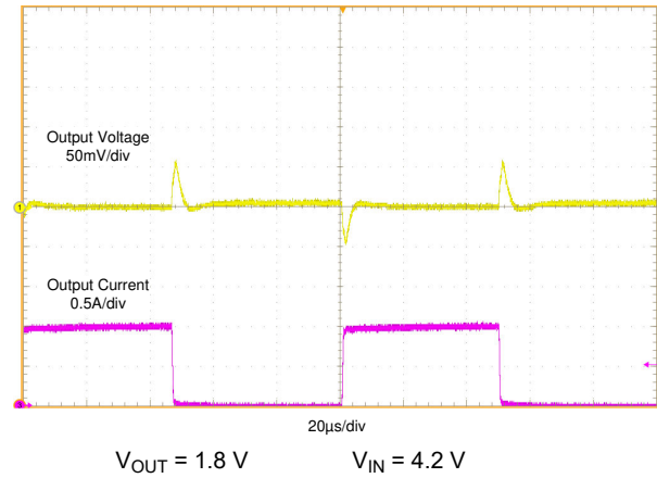
图 8-6. Load Transient In PWM
