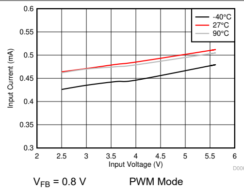
图 6-6. Non-Switching Input Current in PWM Mode
