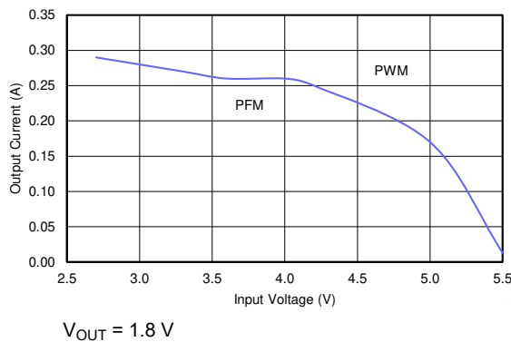
图 8-9. AUTO Mode Thresholds
