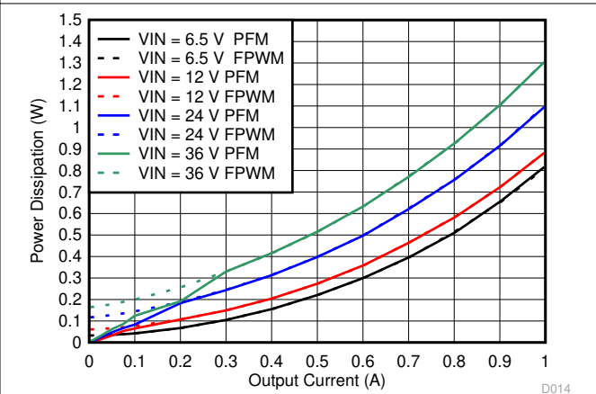
图 6-10. Power Dissipation
