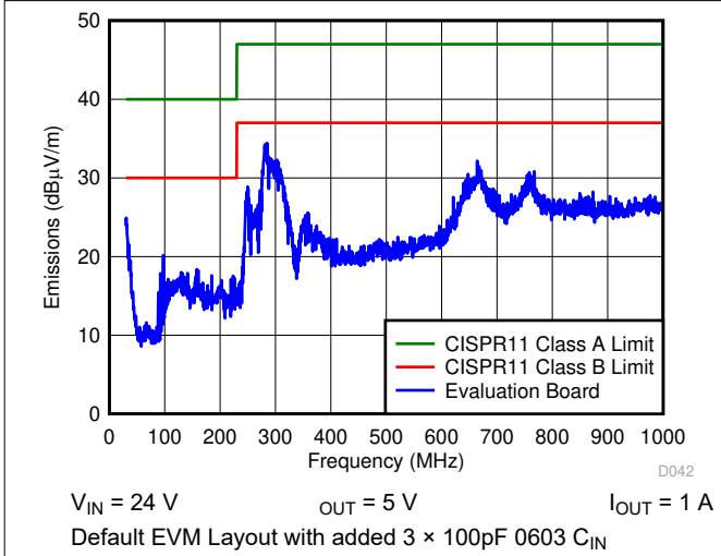
图 6-7. Radiated EMI
