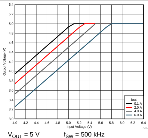
图 41. Voltage Dropout
