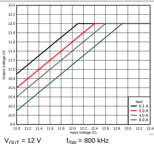
图 43. Voltage Dropout
