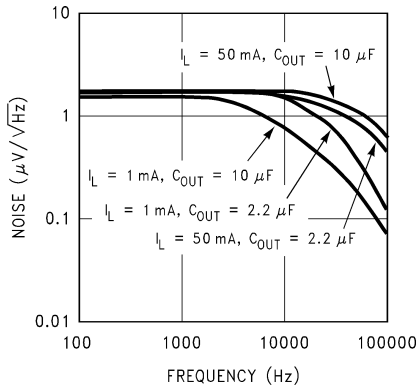
图 5-25. Output Noise Density (Legacy Chip)
