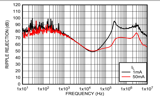
图 5-28. Ripple Rejection (Legacy Chip)
