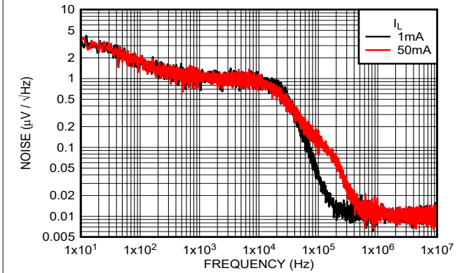
图 5-25. Output Noise Density (Legacy Chip)
