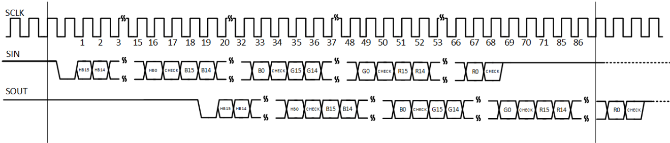
图 6-19. 使用广播的数据写入命令 ( 时序图 )
