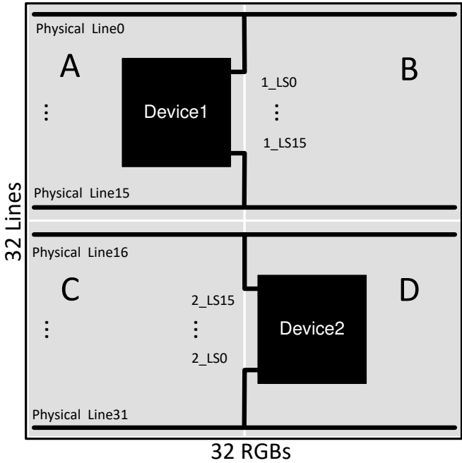
图 6-2. Mode2 示意图
