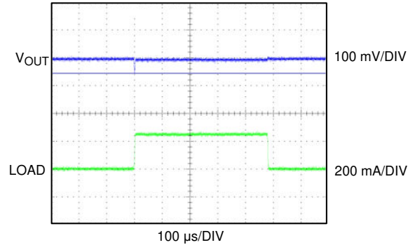
图 5-14. Load Transient
