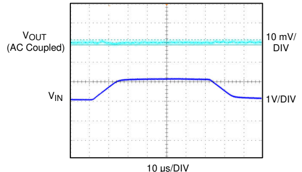
图 5-8. 线路调整
