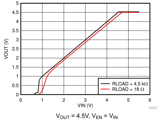
图 5-4. V_{OUT} vs V_{IN}
