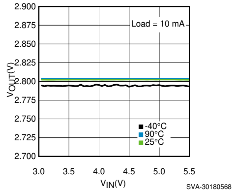
图 5-8. 线路调整
