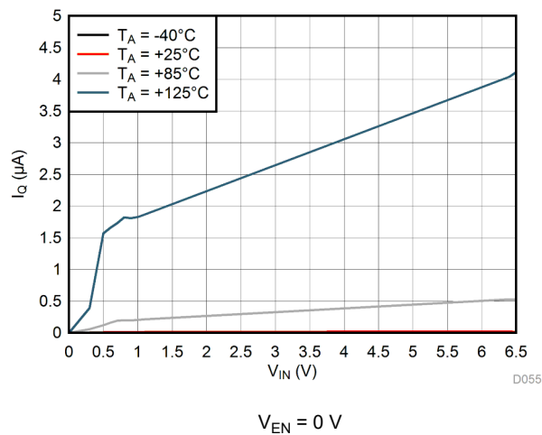
图 6-15. LP5912-1.8 I_{Q(SD)} vs V_{IN}
