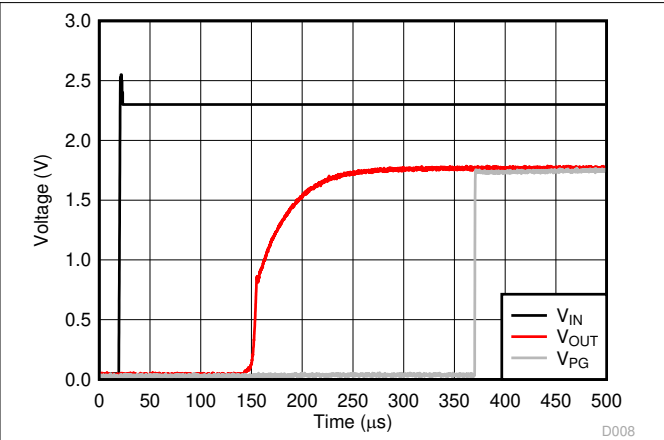
图 6-8. LP5912-1.8 Power Up
