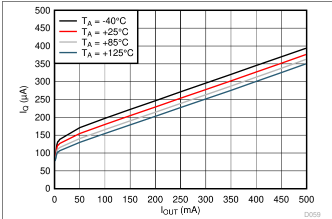
图 6-19. LP5912-3.3 I_{Q(SD)} vs I_{OUT}
