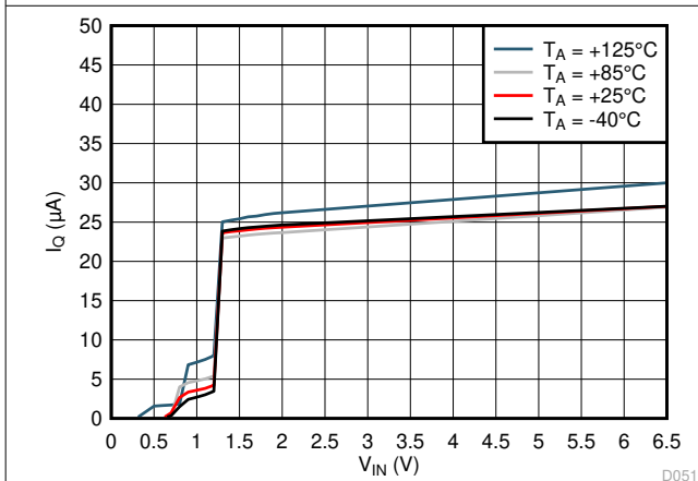
图 6-9. LP5912-3.3 Power Up
