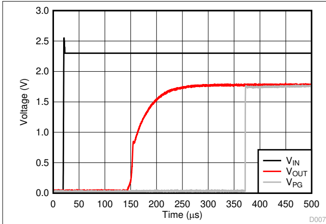
图 6-7. LP5912-1.8 Power Up
