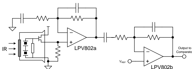
PIR 运动检测器中的毫微功耗放大器
