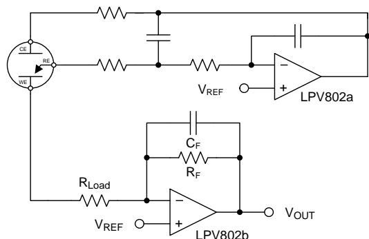
电化学传感器中的毫微功耗放大器
