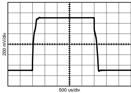
图 27. 小信号脉冲响应, 1.8V
