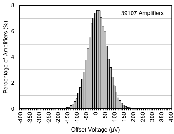
图 3. LPV811 的失调电压分布
