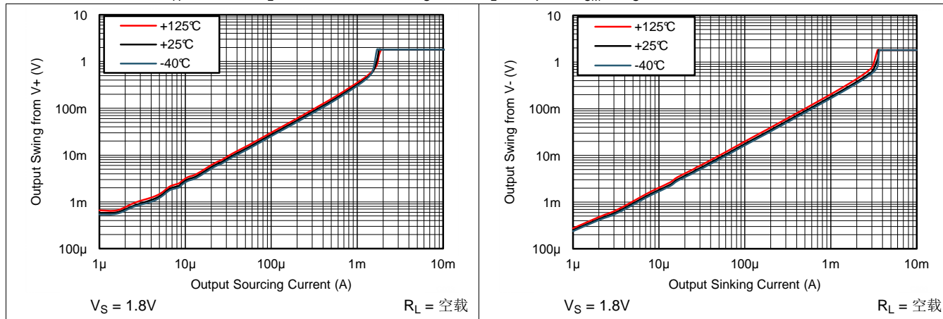
图 21. 输出摆幅与拉电流间的关系, 1.8V
