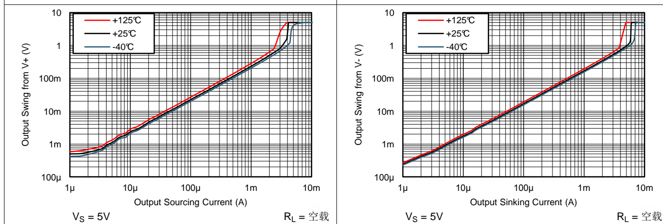
图 25. 输出摆幅与拉电流间的关系, 5V
