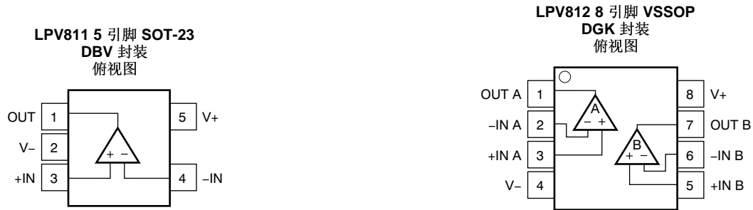
引脚功能: LPV811 DBV
