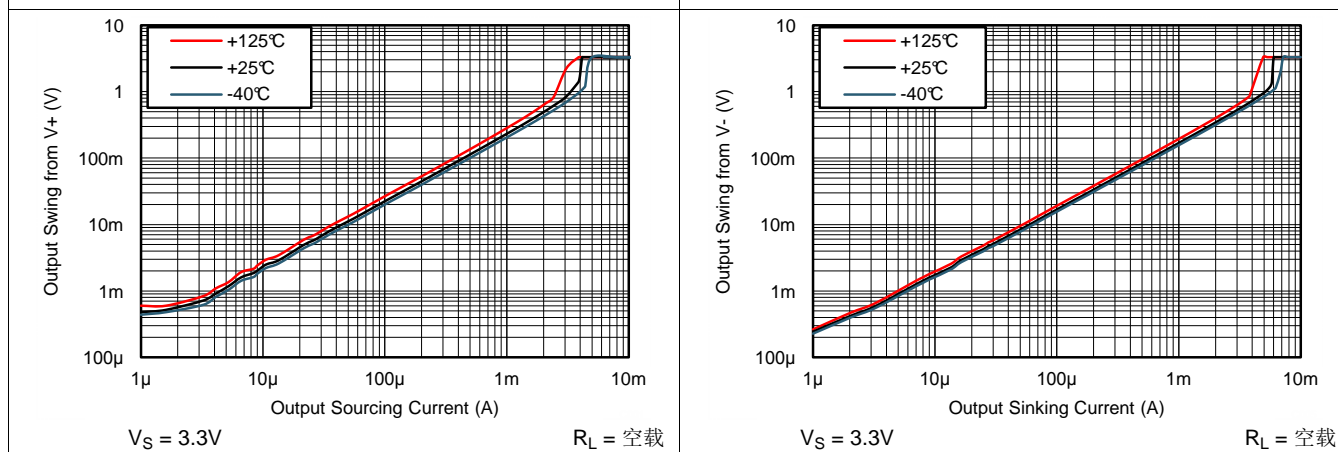
图 23. 输出摆幅与拉电流间的关系, 3.3V
