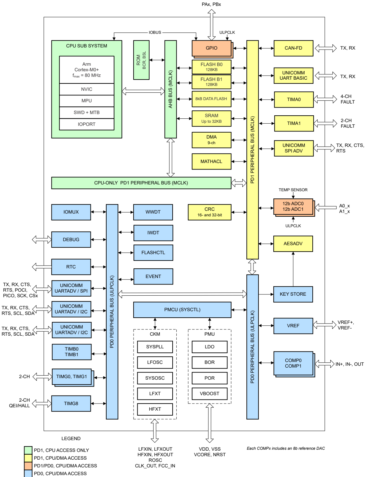
图 4-1. MSPM0G3218-Q1 功能框图
