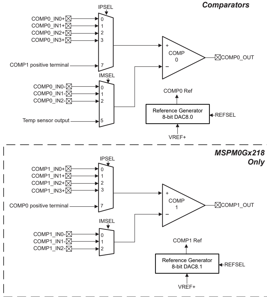
图 8-6. 比较器模拟连接
