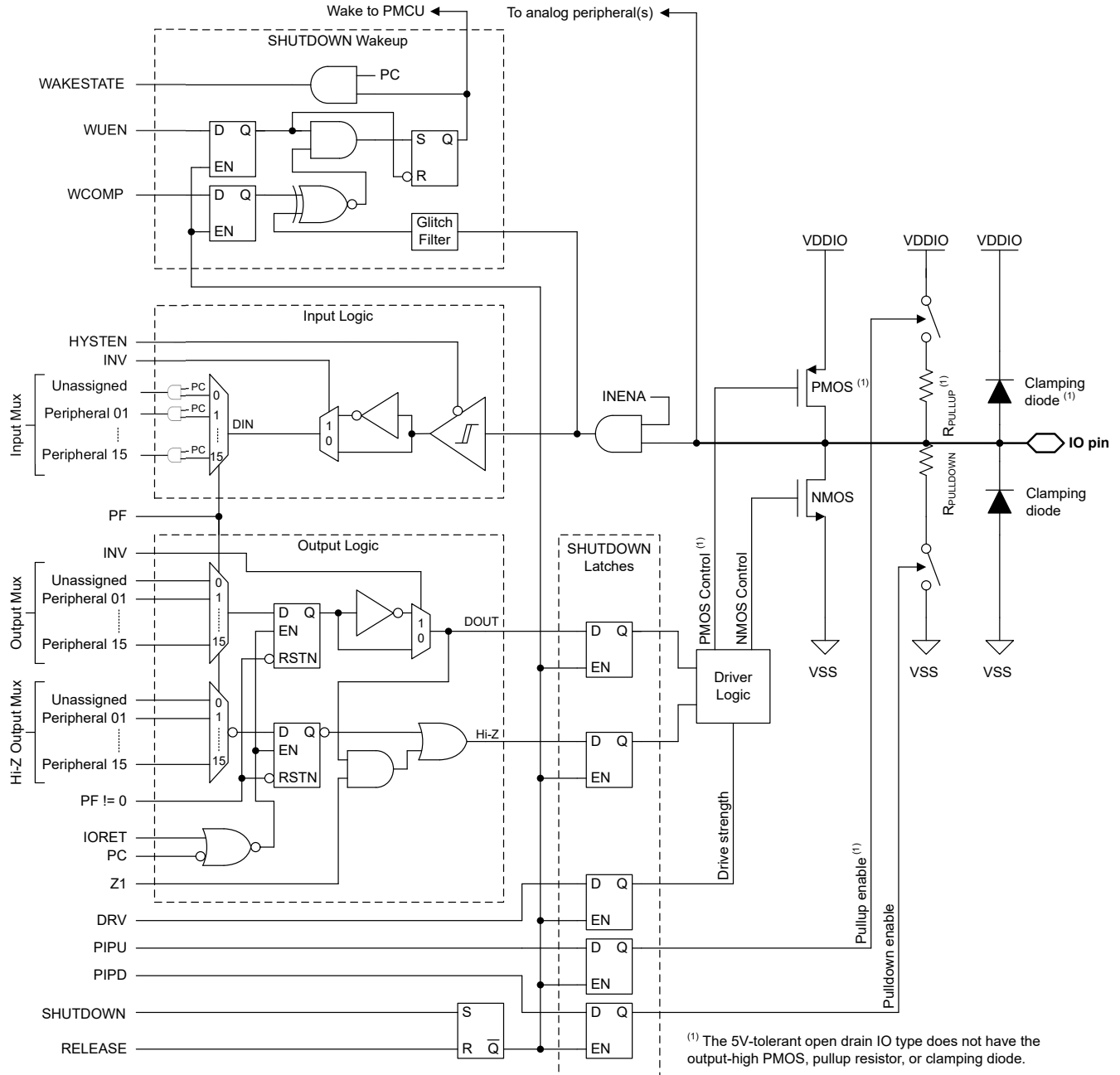
图 8-5. 超集输入/输出图
