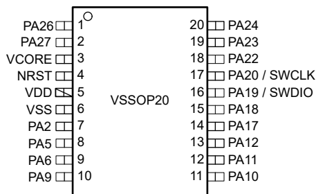
图 6-7. 20 引脚 20DGS (0.5mm) (VSSOP) 封装图
