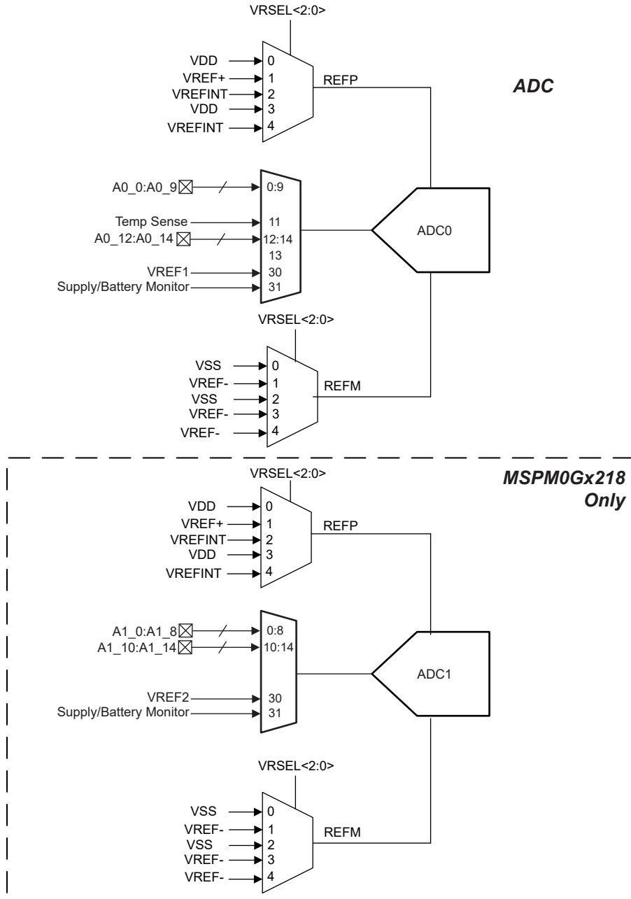
图 8-7. ADC 模拟连接
