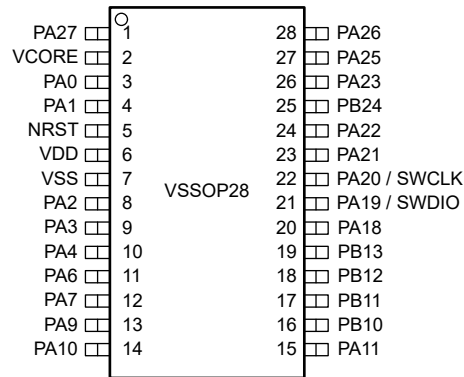
图 6-5. 28 引脚 28DGS (0.5mm) (VSSOP) 封装图
