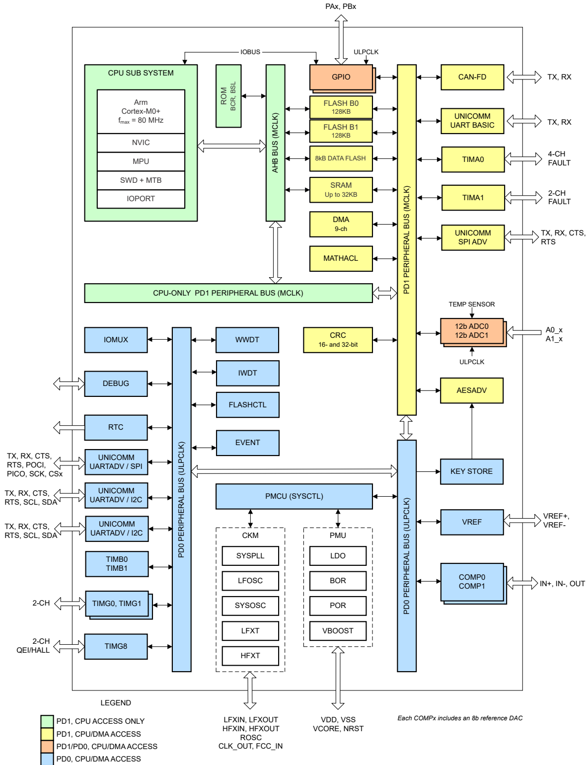
图 8-1. MSPM0G3218-Q1 功能框图
