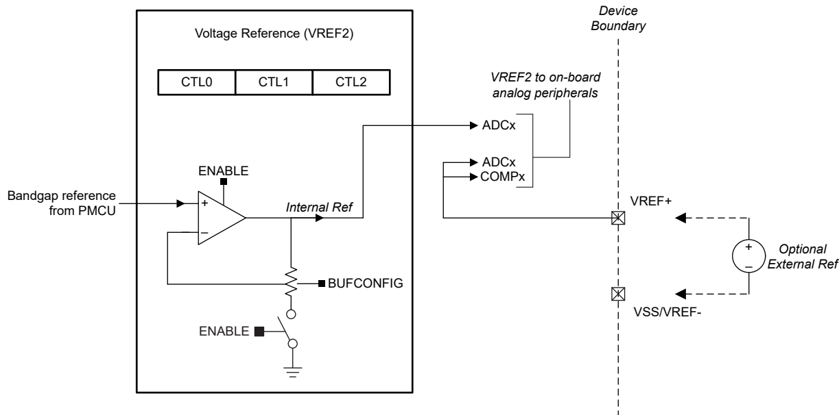
图 8-4. VREF2 (VREFINT) 模块
