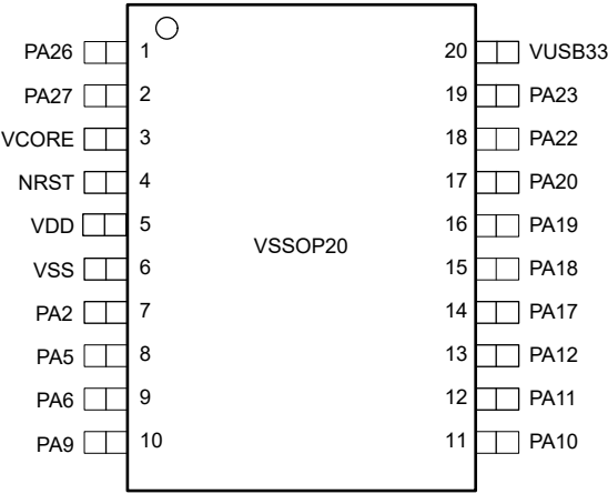
图 6-8. 20 引脚 DGS (0.5mm) (VSSOP) 封装图
