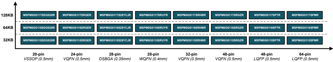
图 5-1. 器件比较图
