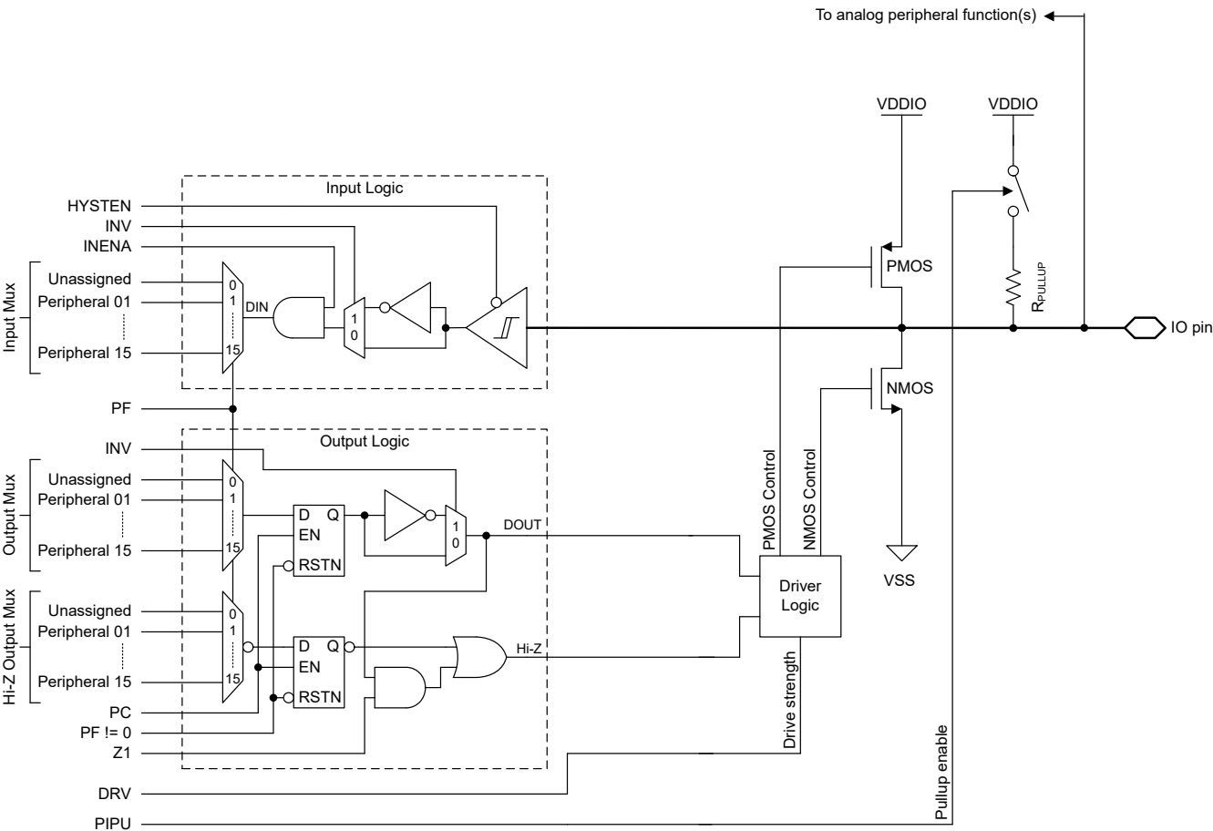
图 8-3. 超集输入/输出图
