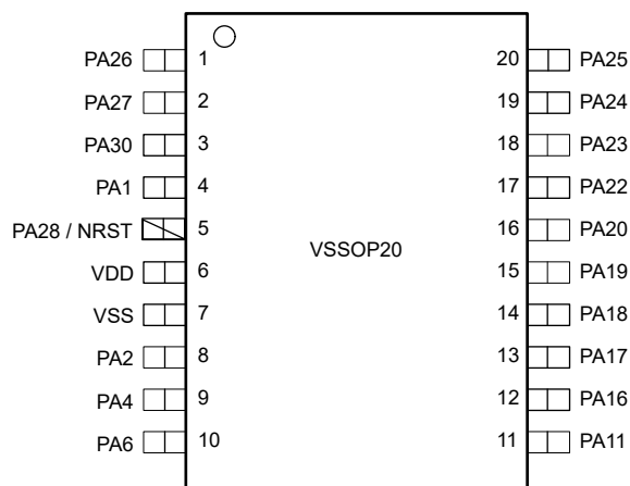
图 6-6. 20 引脚 DGS20 (VSSOP) (顶视图)
