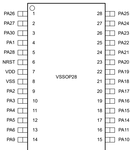
图 6-4. 28 引脚 DGS28 (VSSOP) ( 顶视图 )
