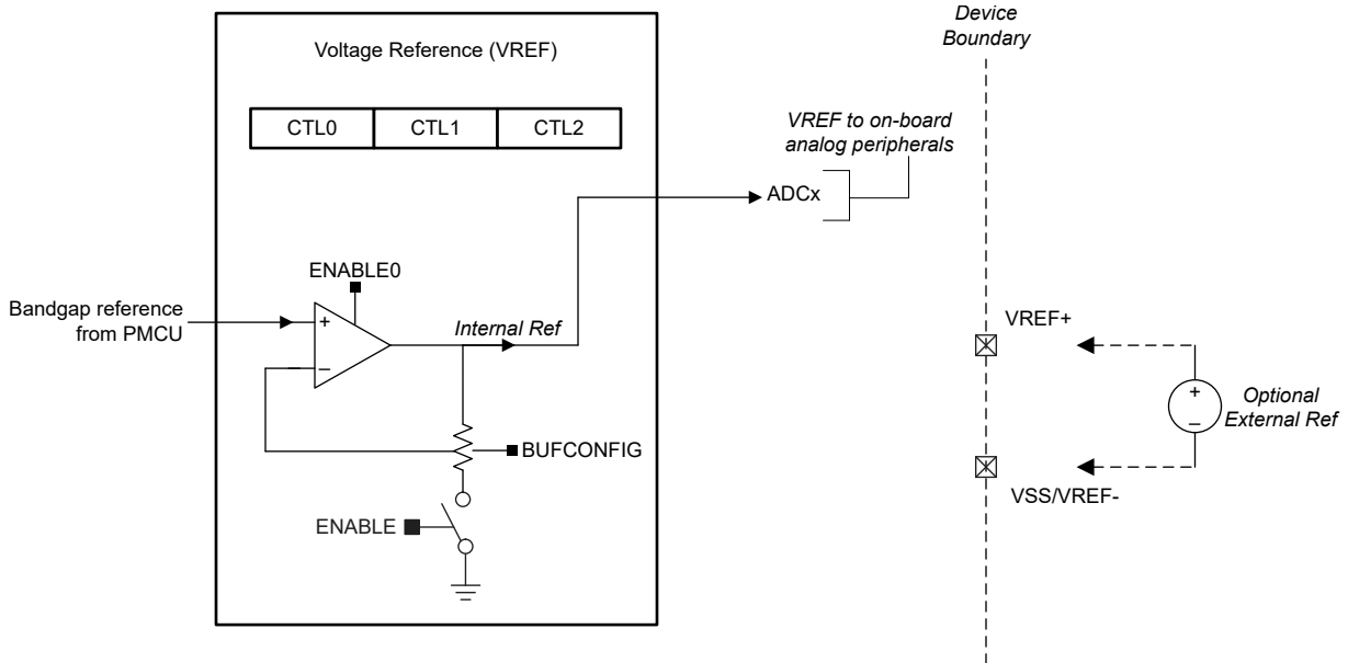
图 8-1. VREF 模块
