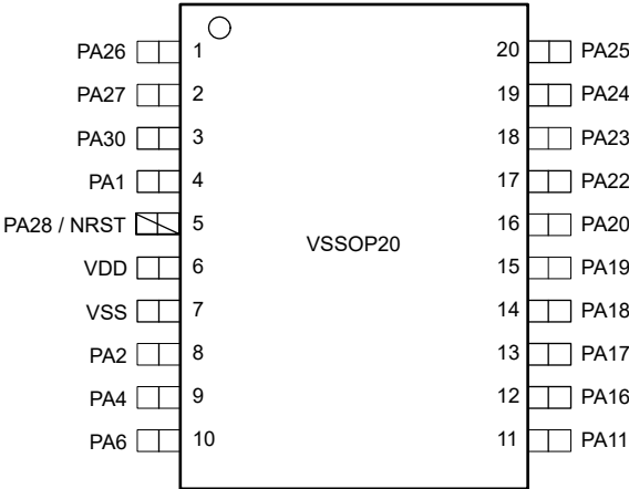
图 6-7. 20 引脚 DGS20 (VSSOP) ( 顶视图 )
