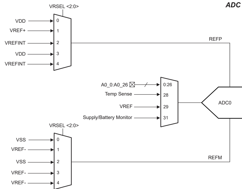
图 8-2. 模拟连接
