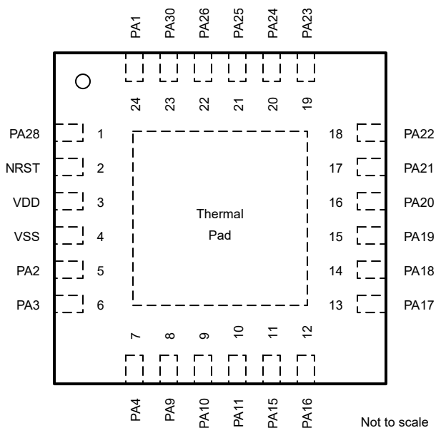
图 6-6. 24 引脚 RGE (VQFN) (顶视图)
