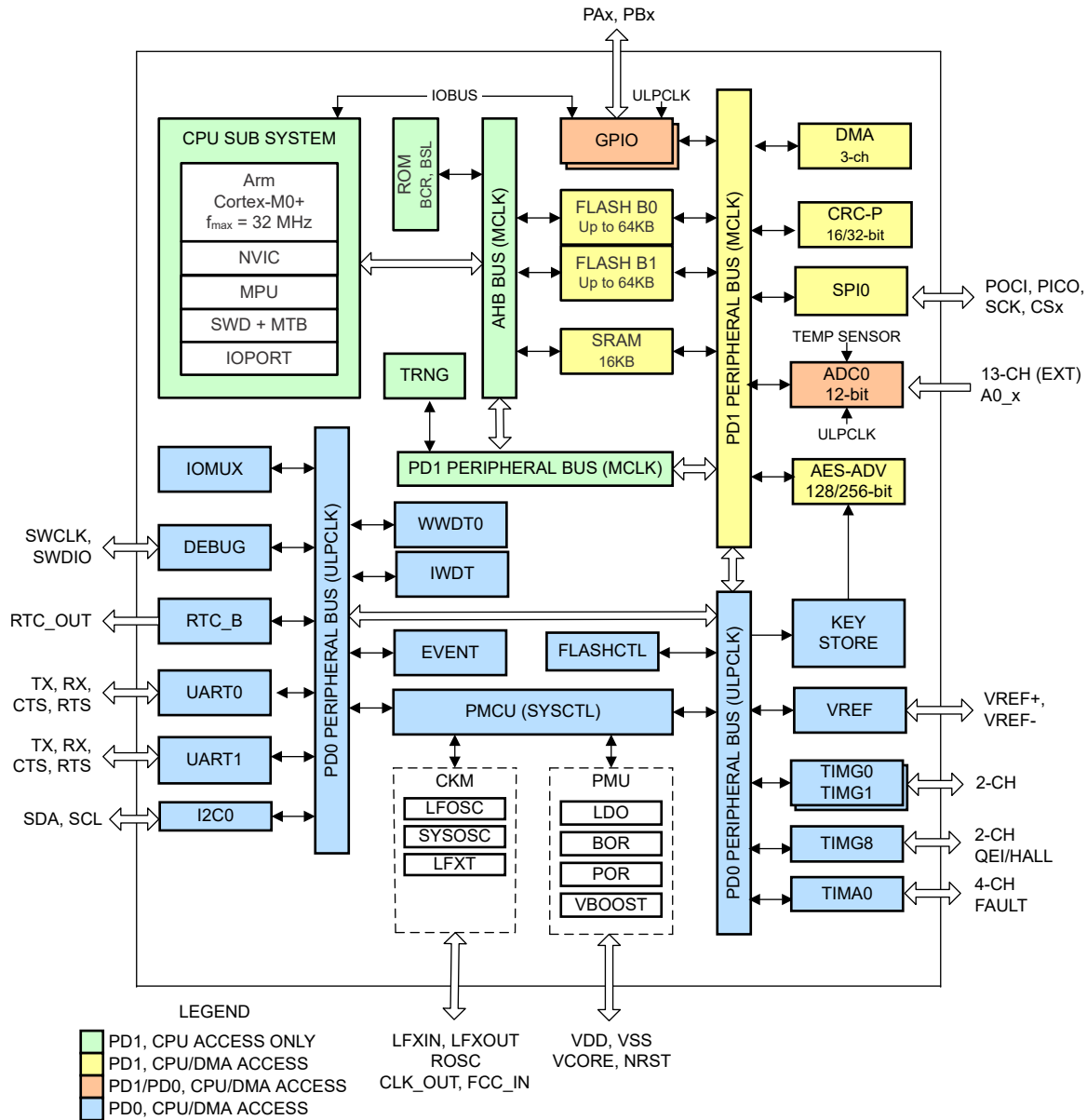
图 4-1. MSPM0L111x-Q1 功能方框图
