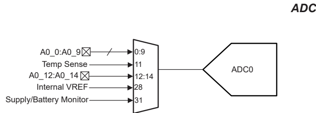
图 8-2. 模拟连接
