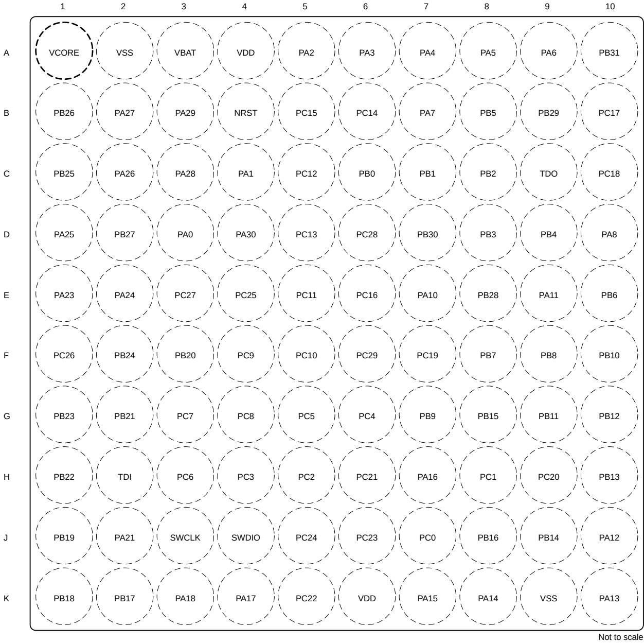
图 6-1. 100 引脚 ZAW (0.8mm) (NFBGA) 封装图 ( 顶视图 )
