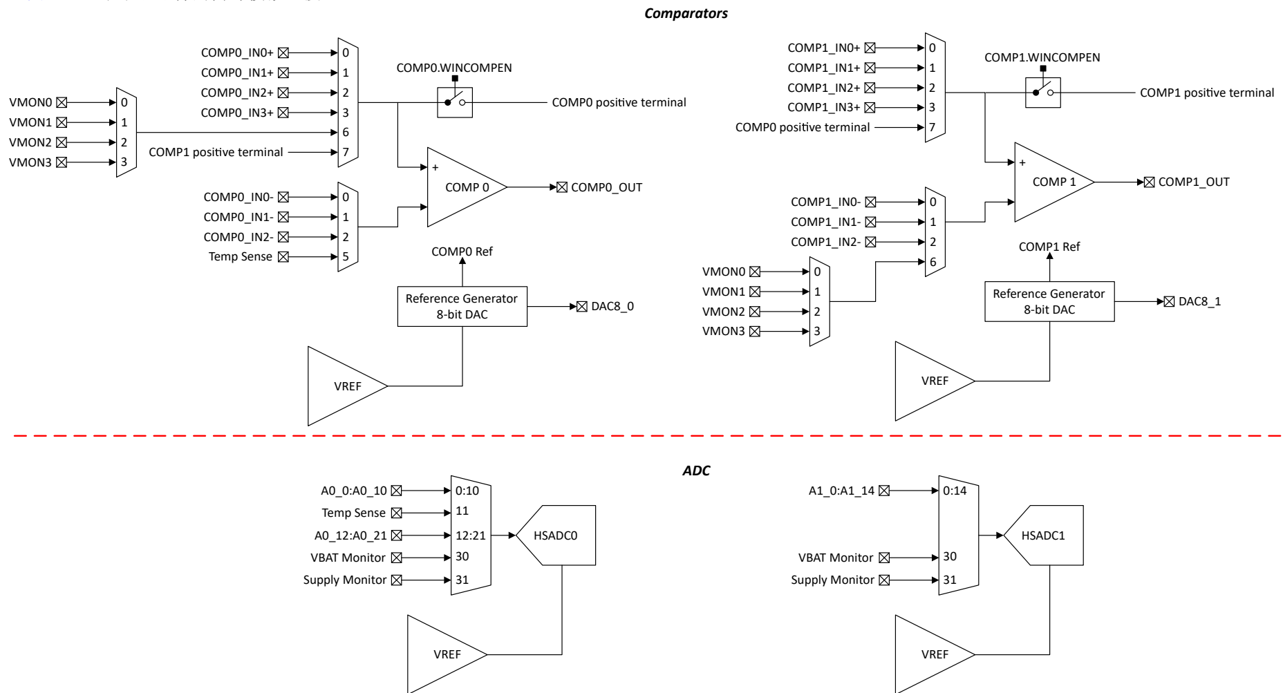
图 8-2. 器件模拟连接
