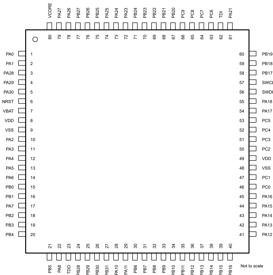
图 6-3. 80 引脚 PN (0.5mm) (LQFP) 封装 ( 顶视图 )
