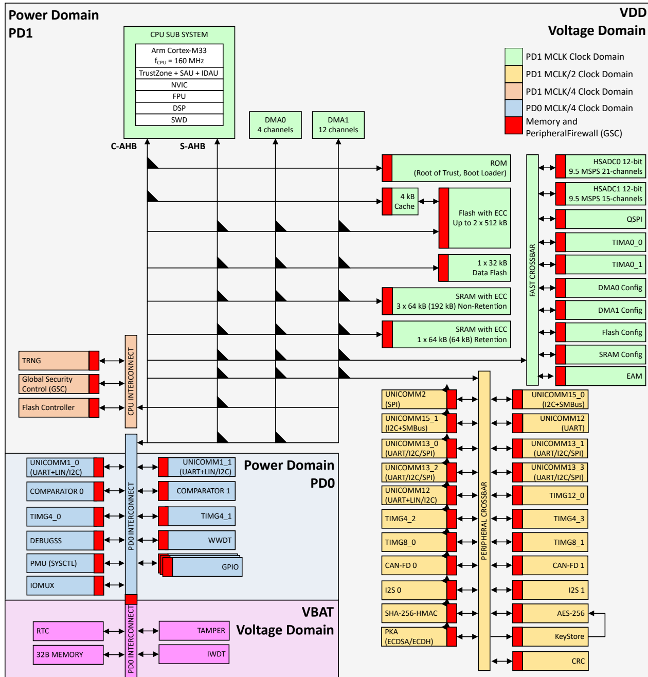
图 4-1. MSPM33C321x 功能方框图
