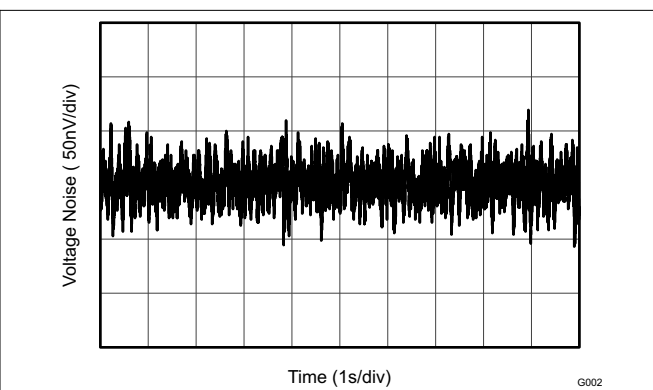
图 5-2. 0.1Hz 至 10Hz 噪声
