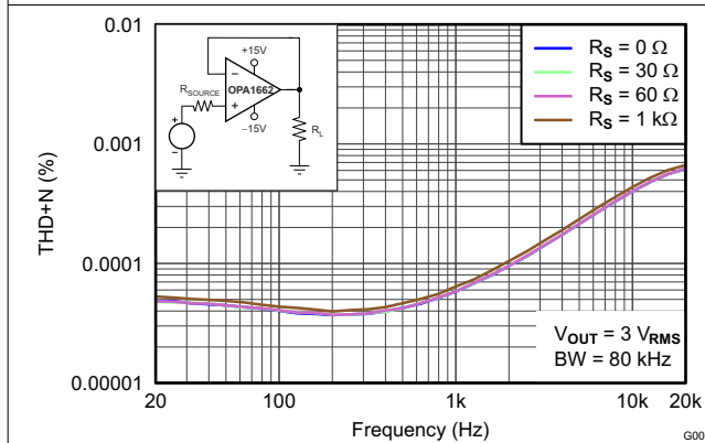
图 5-9. THD+N 比与频率间的关系
