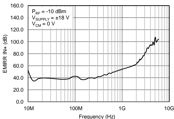
图 57. EMIRR 测试
