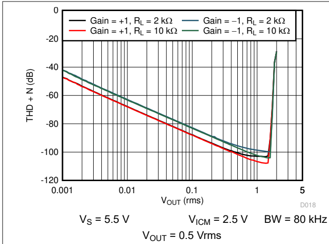
图 7-19. THD + N vs Amplitude
