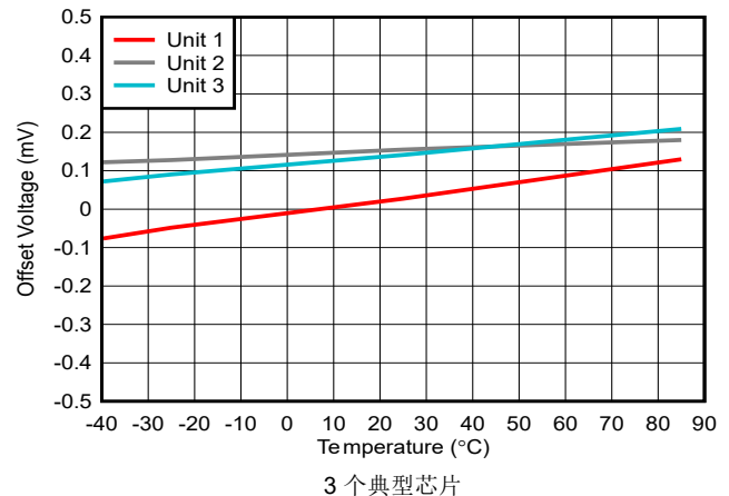
图 5-24. 输入失调电压与环境温度间的关系
