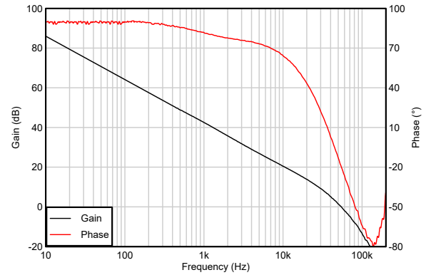
图 5-10. 开环增益和相位与频率间的关系
