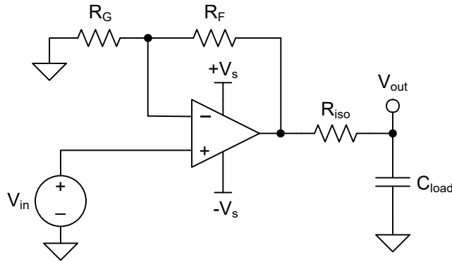
图 6-3. 增强容性负载驱动能力
