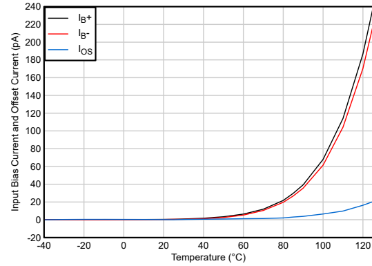
图 5-8. I_B 和 I_{OS} 与温度间的关系
