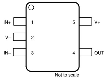
图 4-2. OPA371D DCK 封装 5 引脚 SC70 顶视图
