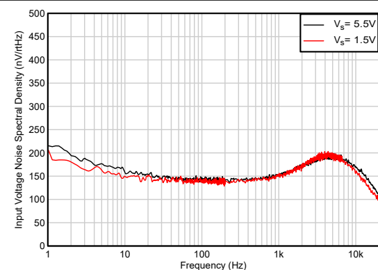
图 5-24. 输入电压噪声频谱密度
