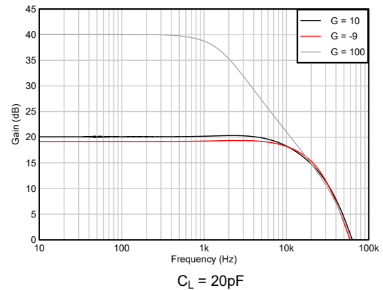
图 5-12. 闭环增益与频率间的关系
