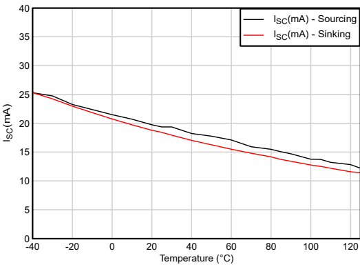
图 5-38. 短路电流与温度间的关系 ( V_S = 5.5\text{V} )
