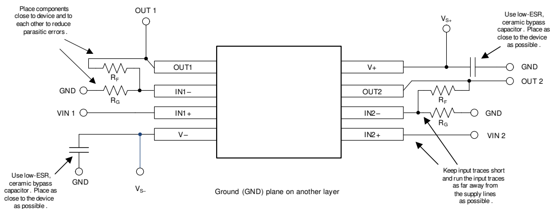
图 7-4. 布局示例
