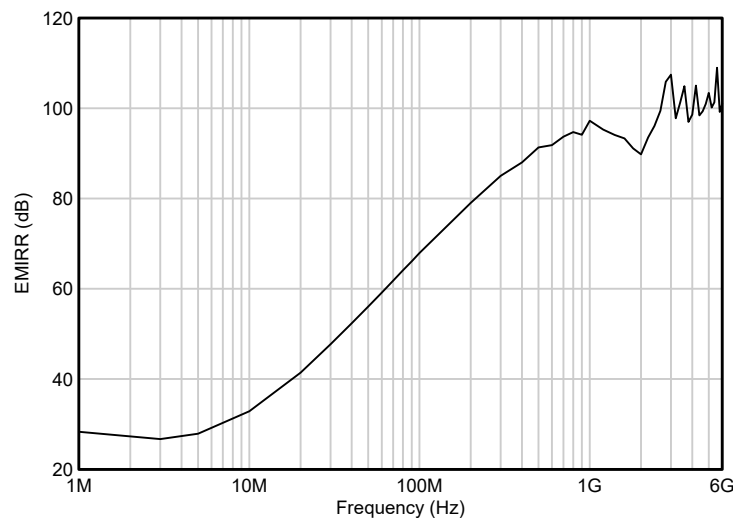
图 6-4. EMIRR 测试
