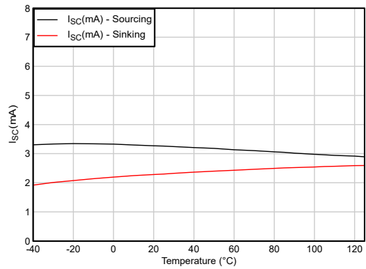
图 5-39. 短路电流与温度间的关系 ( V_S = 1.5\text{V} )
