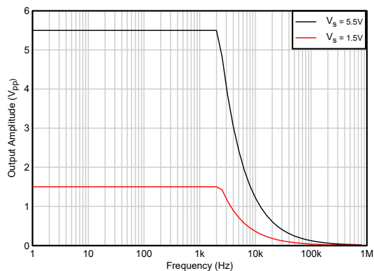
图 5-17. 最大输出电压与频率间的关系
