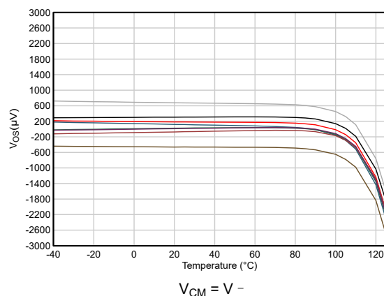
图 5-4. 输入失调电压与温度间的关系
