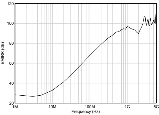
图 5-40. EMIRR 与频率间的关系
