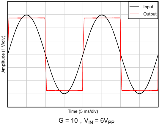
图 5-37. 无相位反转
