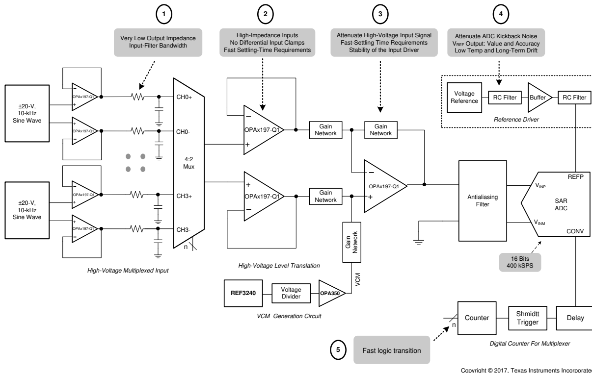
图 8-1. OP Ax197-Q1 在 16 位、400-kSPS、4 通道、多路复用数据采集系统中用于高电压输入，具有最低失真
