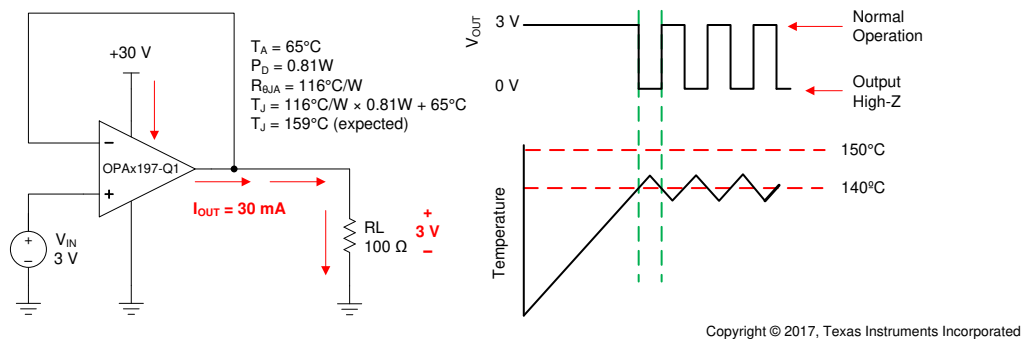
图 7-6. Thermal Protection
