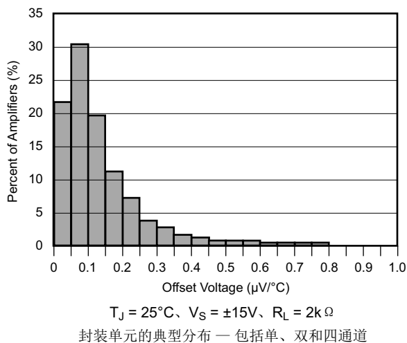
图 7-2. 预热失调电压温漂
