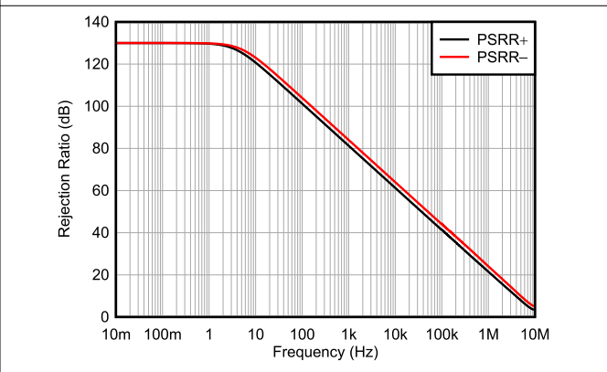
图 6-16. PSRR vs Frequency
