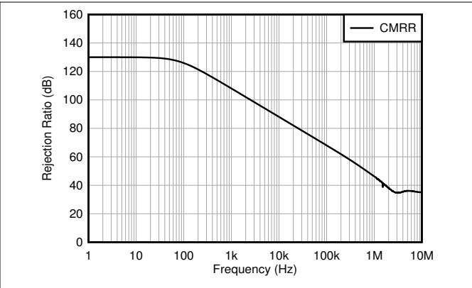
图 6-14. CMRR vs Frequency
