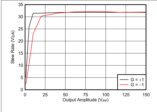
图 6-43. Slew Rate vs Output Step Size
