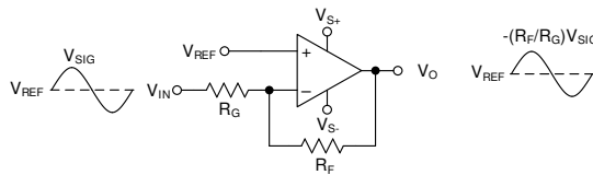
图 8-4. Inverting Amplifier
