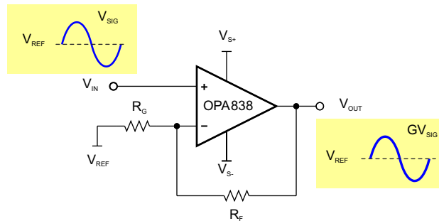
图 7-1. Noninverting Amplifier
