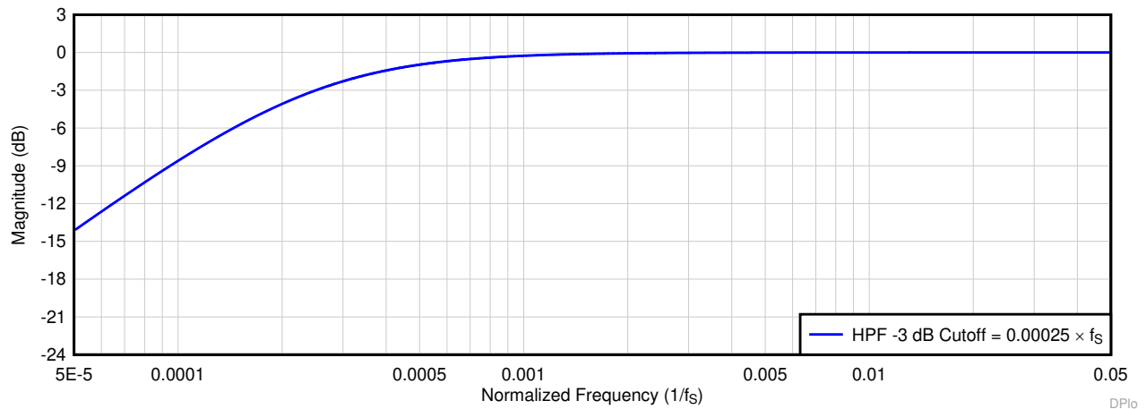
图 6-10. HPF 滤波器频率响应图
