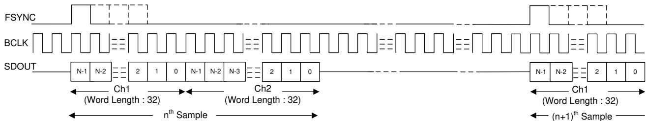
图 6-2. 目标模式下的 TDM 模式协议时序 (FMT0 = 高电平)
