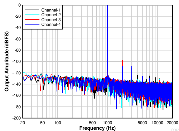
图 6-16. 输入为 -1dBm 时的 FFT
