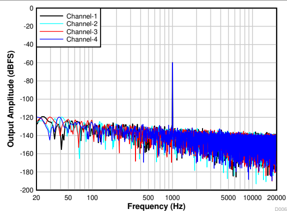
图 6-15. 输入为 -60dBm 时的 FFT
