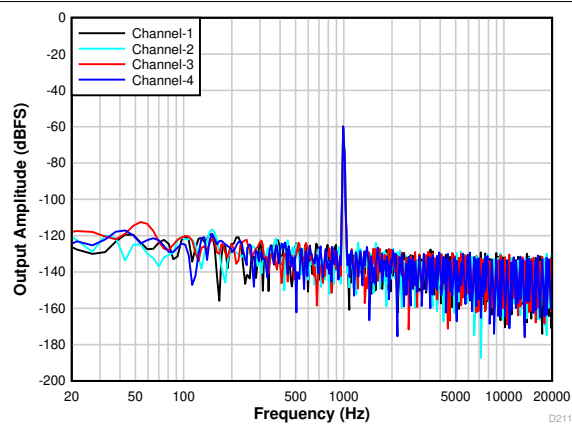
图 9-2. 具有 -60dB 输入的 FFT
