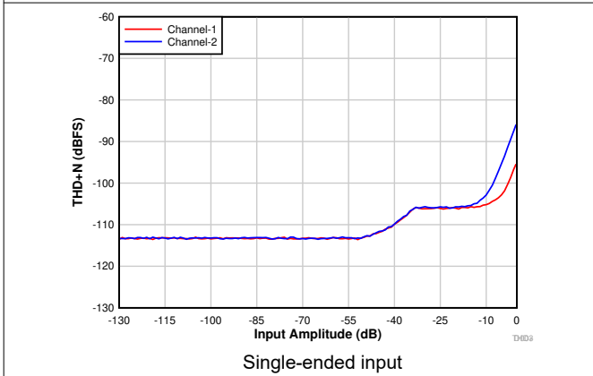
图 7-6. THD+N vs Input Amplitude With DRE Enabled
