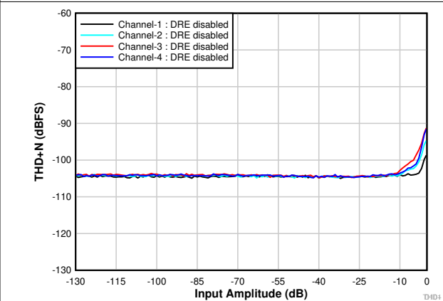
图 6-8. THD+N 与输入幅度间的关系 (DRE 已禁用)
