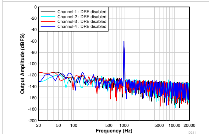
图 8-4. 具有 -60dB r 输入的 FFT (DRE 已禁用)
