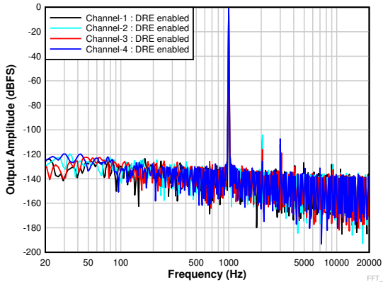
图 6-21. 输入为 -1dBm 时的 FFT (DRE 已启用)
