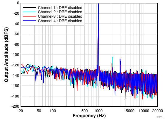
图 6-22. 具有 -1dBm 输入的 FFT (DRE 已禁用)
