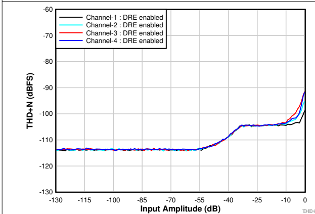
图 6-7. THD+N 与输入幅度间的关系 (DRE 已启用)
