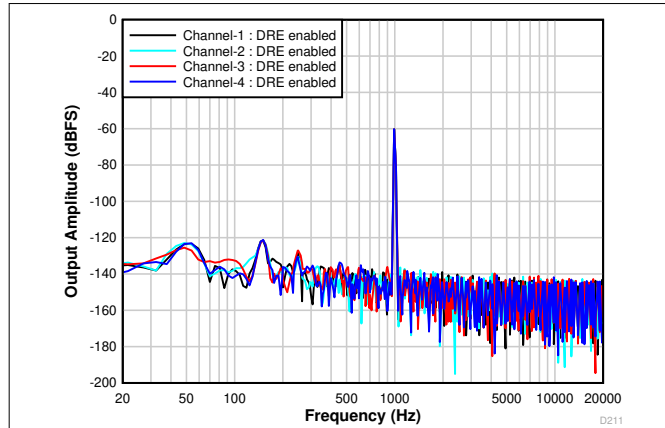
图 8-2. 具有 -60dB r 输入的 FFT (DRE 已启用)
