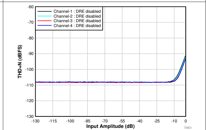
图 8-5. THD+N 与输入幅度间的关系 (DRE 已禁用)
