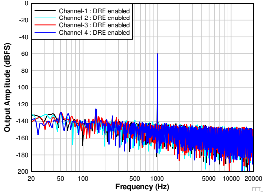
图 6-19. 输入为 -60dBm 时的 FFT (DRE 已启用)
