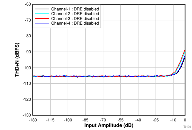
图 6-6. THD+N 与输入幅度间的关系 (DRE 已禁用)
