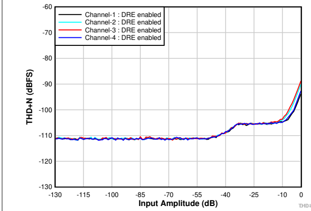
图 6-5. THD+N 与输入幅度间的关系 (DRE 已启用)
