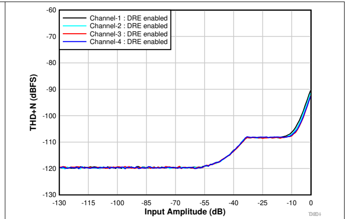
图 8-3. THD+N 与输入幅度间的关系 (DRE 已启用)
