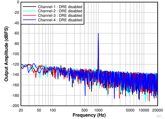
图 6-20. 具有 -60dBm 输入的 FFT (DRE 已禁用)
