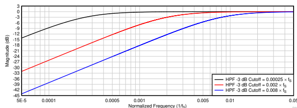
图 6-17. HPF 滤波器频率响应图
