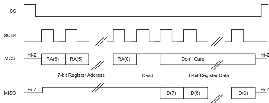
图 6-69. SPI 单字节读取传输
