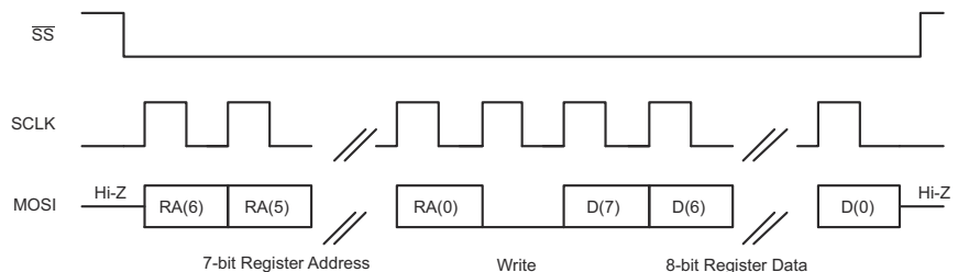
图 6-68. SPI 单字节写入传输
