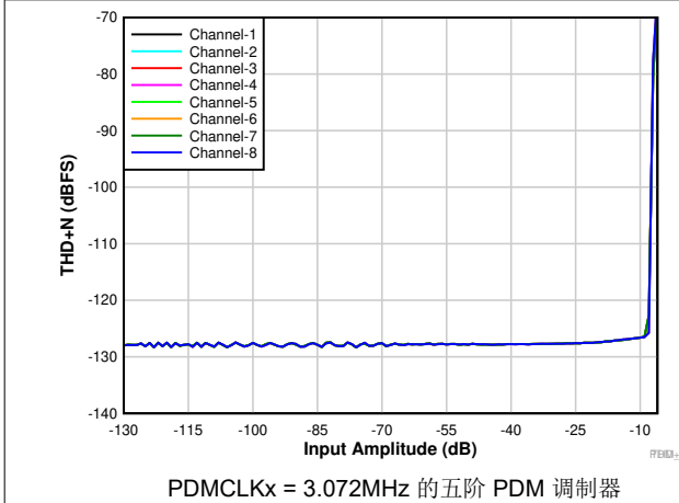
图 5-5. THD+N 与输入幅度间的关系
