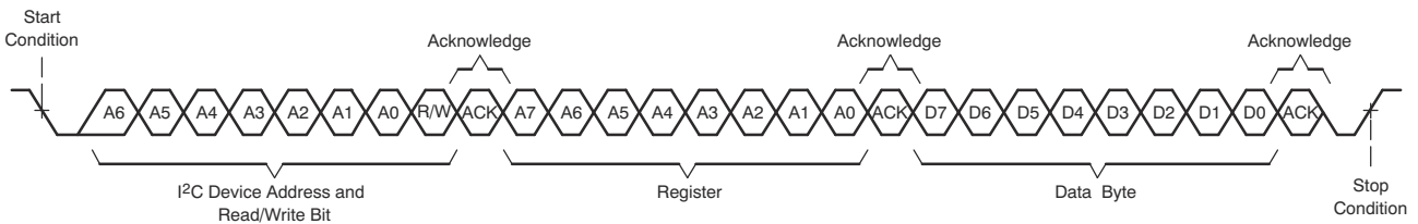
图 6-64. I 2 C 单字节写入传输
