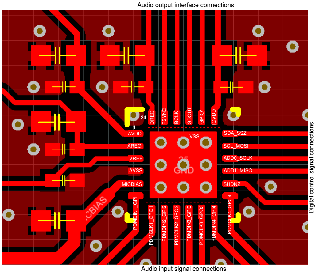
图 10-1. 布局示例
