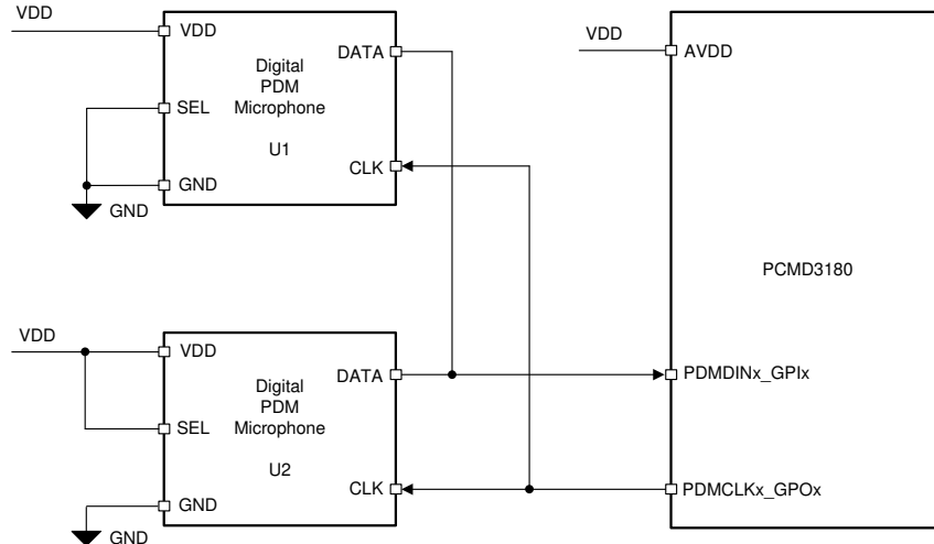
图 6-14. 数字 PDM 麦克风与 PCMD3180-Q1 的连接图
