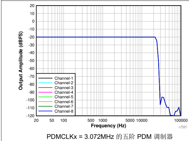
图 5-7. 输入为 -20dB 时的频率响应
