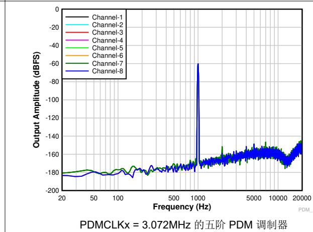
图 5-8. 输入为 -60dB 时的 FFT
