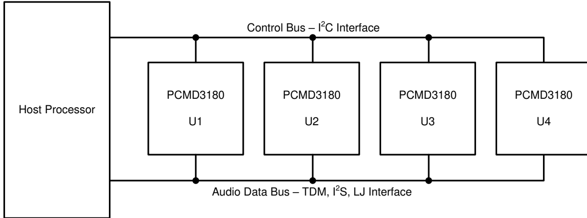
图 6-13. 多个 PCMD3180-Q1 器件具有共享控制和音频数据总线
