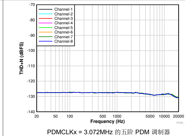
图 5-6. 输入为 -20dB 时 THD+N 与输入频率间的关系
