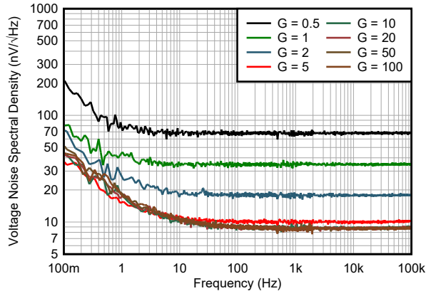
图 6-27. 电压噪声频谱密度 (RTI) 与频率间的关系
