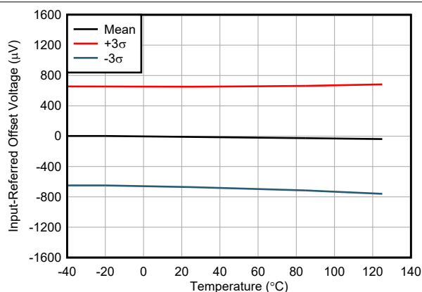
图 6-7. 失调电压 (RTI) 与温度间的关系
