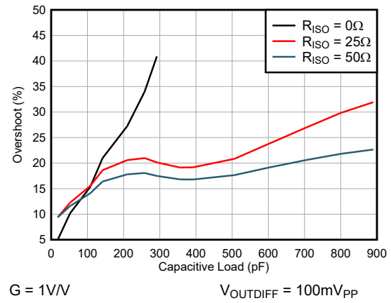
图 6-56. 过冲与容性负载间的关系
