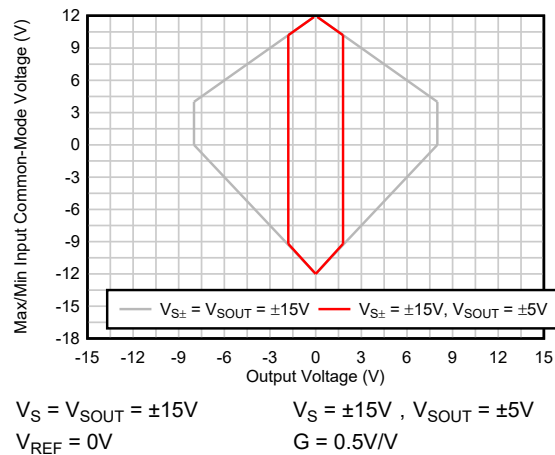
图 8-1. 输入共模电压与输出电压间的关系
