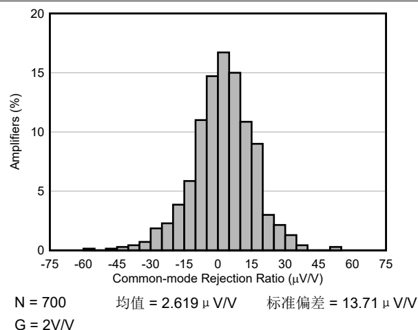
图 6-16. CMRR 分布
