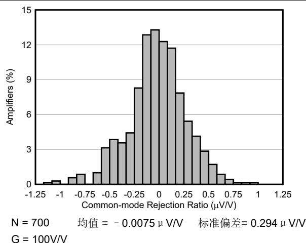
图 6-15. CMRR 分布
