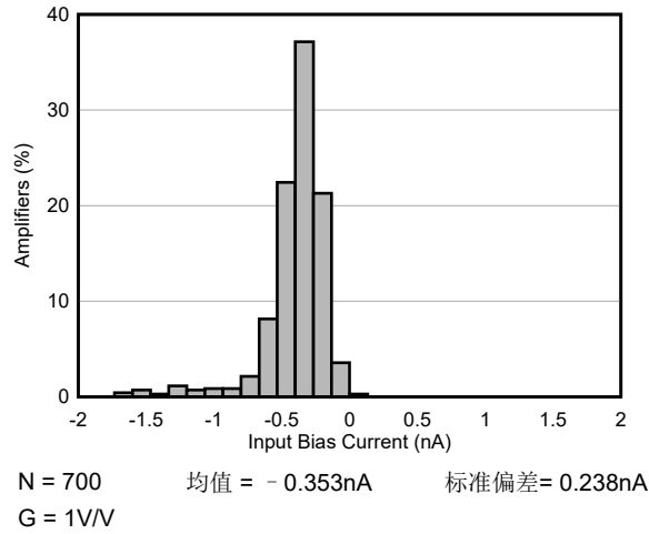
图 6-21. 输入偏置电流的分布
