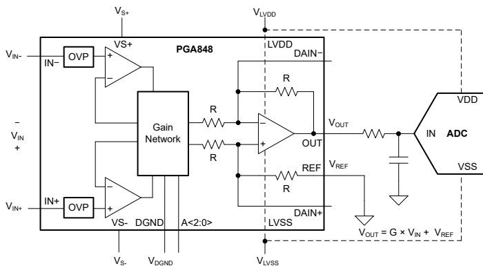
PGA848 简化版应用
