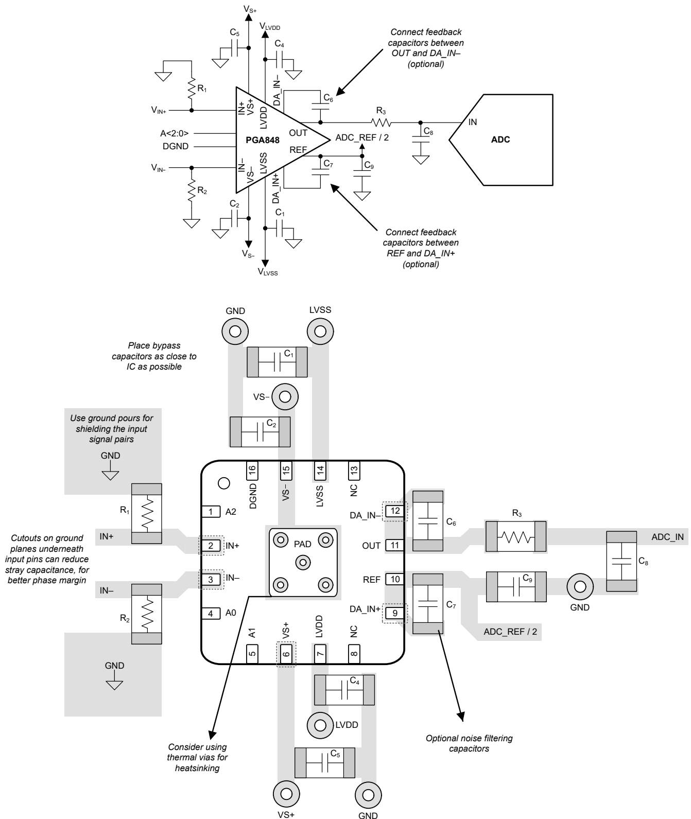
图 8-10. 原理图和相关 PCB 布局示例
