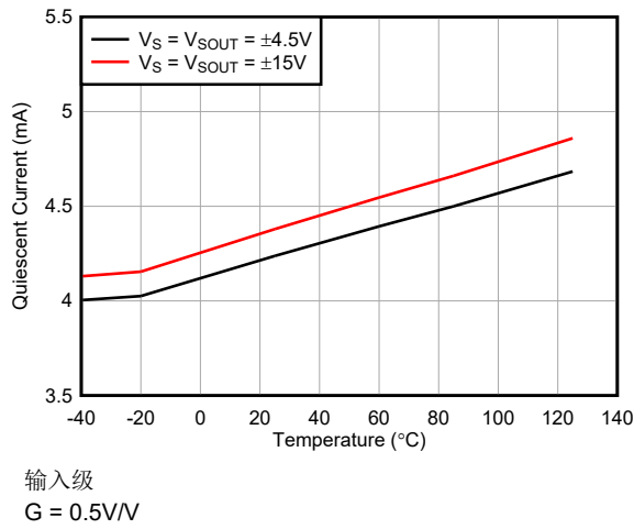
图 6-57. 静态电流与温度间的关系
