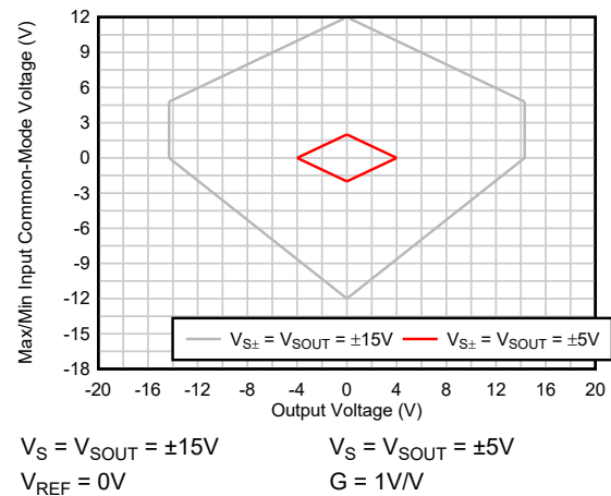
图 8-2. 输入共模电压与输出电压间的关系
