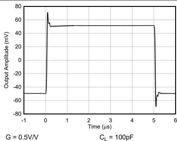
图 6-49. 小信号阶跃响应
