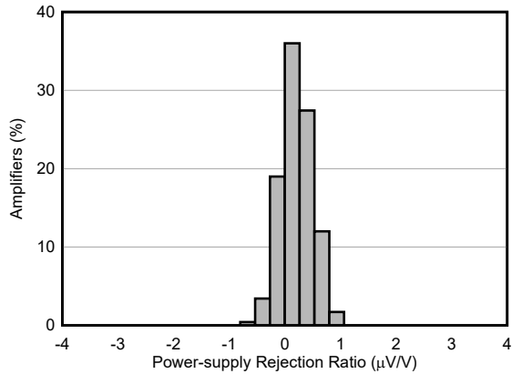
图 6-11. PSRR 分布
