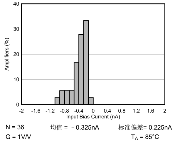
图 6-22. 输入偏置电流的分布
