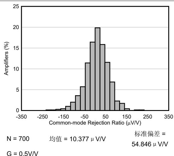
图 6-17. CMRR 分布
