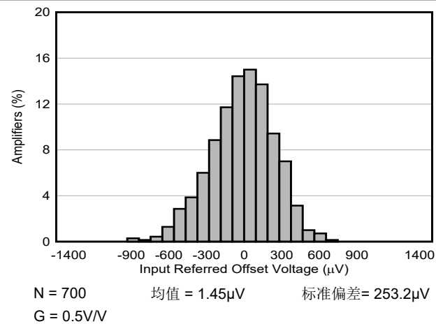
图 6-5. 失调电压 (RTI) 的分布
