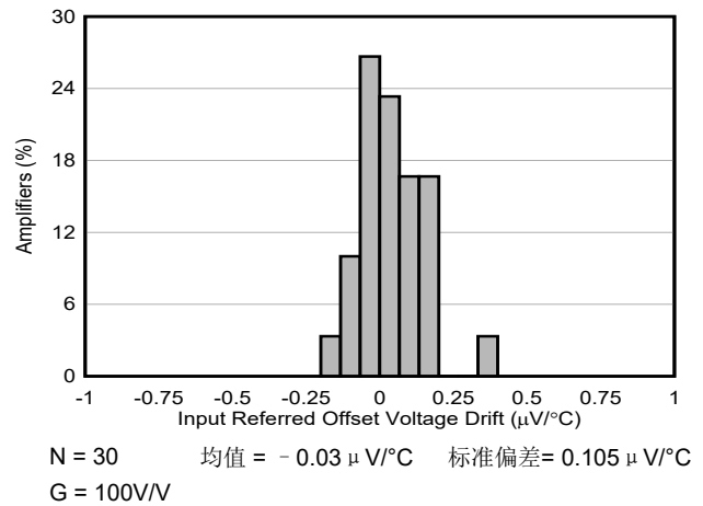
图 6-2. 失调电压漂移 (RTI) 的分布
