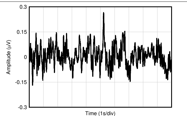
图 5-6. 0.1Hz to 10Hz Noise
