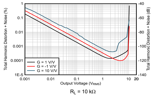
图 5-10. THD+N vs Amplitude
