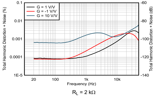
图 5-7. THD+N vs Frequency
