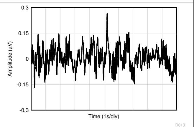
图 5-6. 0.1Hz to 10Hz Noise
