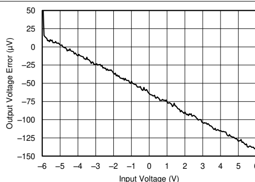
图 9-3. \pm 6\text{V} 输入下测得的输出误差
