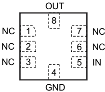
图 5-2. REF3312、REF3318、REF3320、REF3325、 REF3330、REF3333RSE 封装 UQFN-8 (顶视图)
