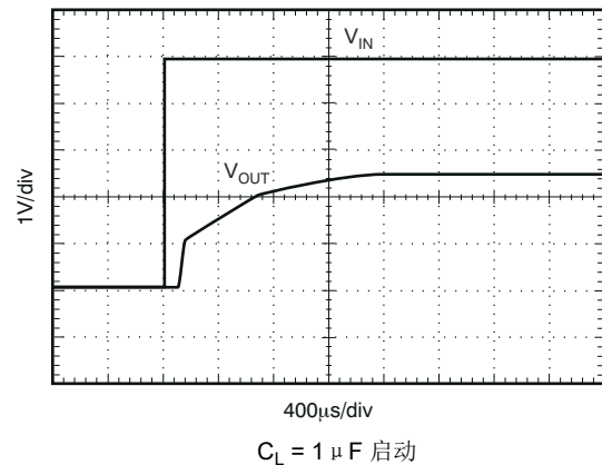
图 6-10. 阶跃响应
