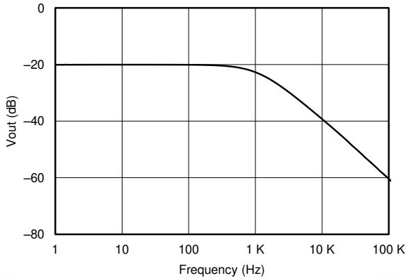
图 9-5. 测得的交流传递函数
