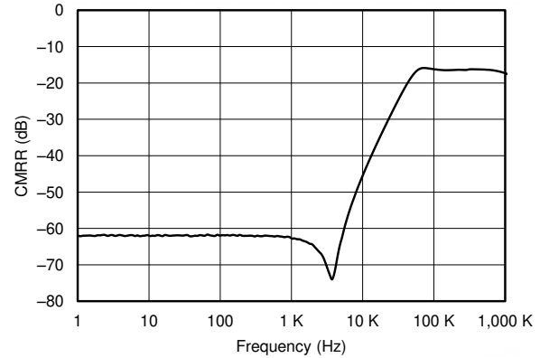
图 9-6. 测得的交流 CMRR 结果
