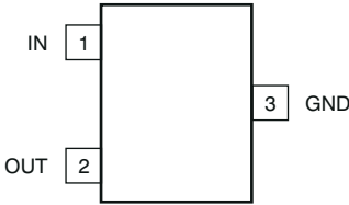
图 5-1. REF3312、REF3318、REF3320、REF3325、 REF3330、REF3333DBZ 封装和 DCK 封装 SOT-23-3、SC70-3 (顶视图)
