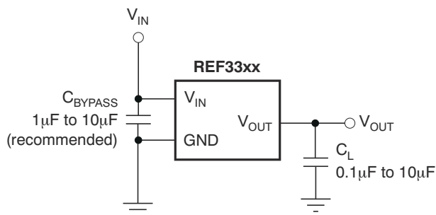
图 8-1. 基本连接
