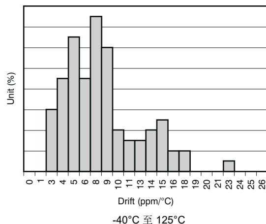
图 6-2. 温漂
