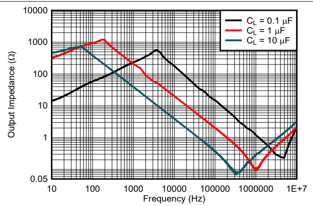
图 6-32. Output Impedance
