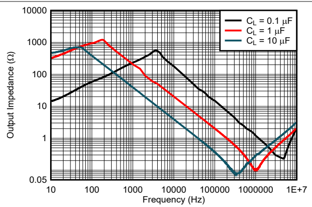
图 6-32. Output Impedance
