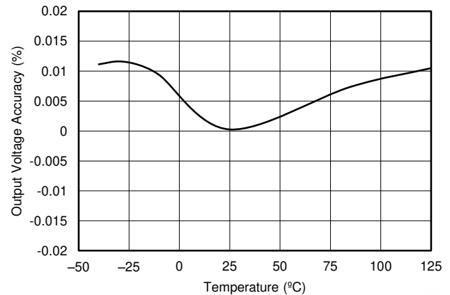
图 6-4. 输出电压精度与温度间的关系
