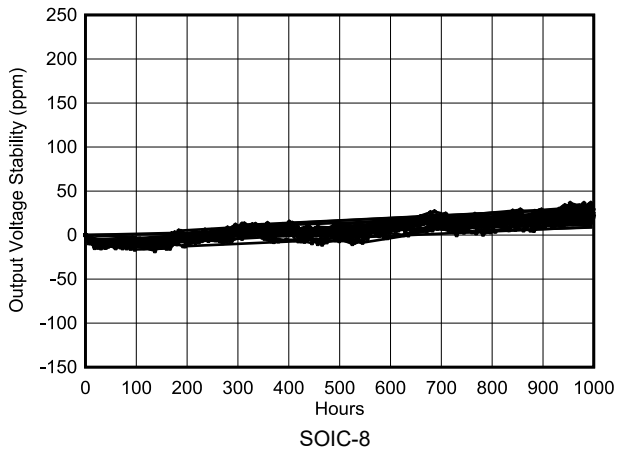
图 6-28. REF50xx 长期稳定性 (前 1000 小时)
