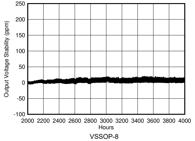
图 6-26. REF50xx 长期稳定性 (后 2000 小时)
