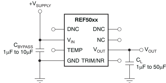
图 8-6. 基本连接
