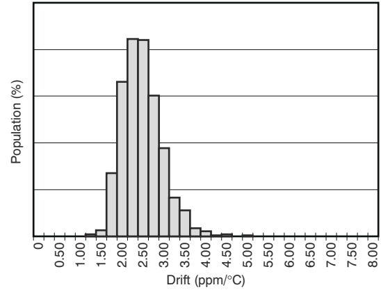
-40°C 至 125°C 图 6-2. 温漂
