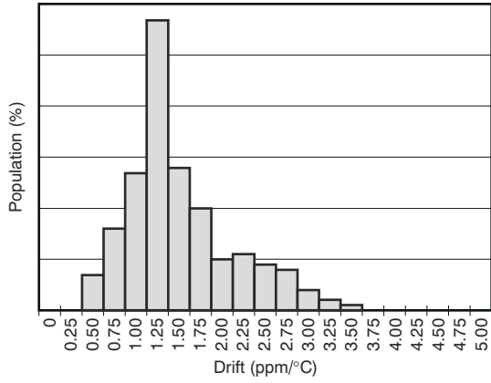
0°C 至 85°C 图 6-1. 温漂
