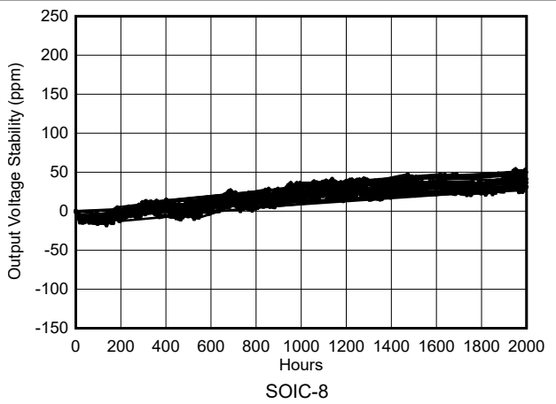
图 6-30. REF50xx 长期稳定性 (2000 小时)
