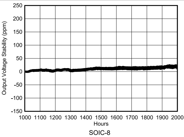
图 6-29. REF50xx 长期稳定性 (后 1000 小时)
