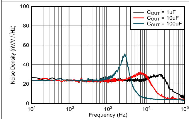
图 6-15. 噪声性能 10Hz 至 100kHz ( C_{NR} = \text{开路} )
