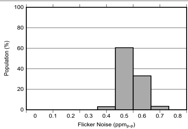
图 6-14. 0.1Hz 至 10Hz 电压噪声分布 ( C_{NR} = \text{开路} )
