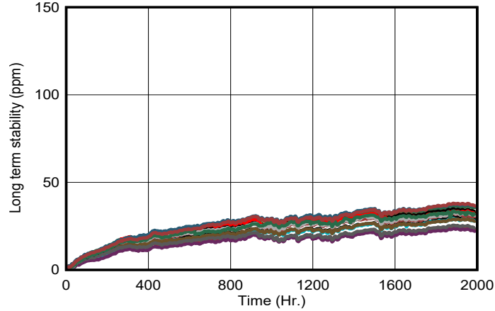
图 7-2. 长期稳定性 SOIC - 2000 小时 ( V_{OUT} )
