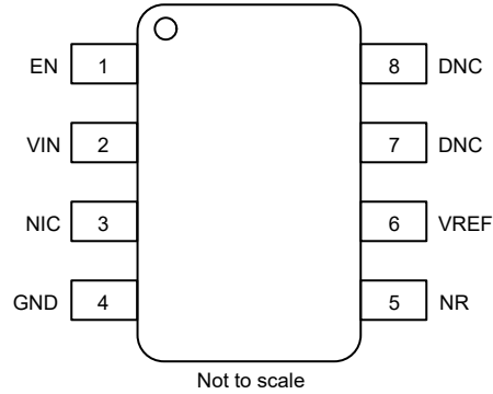
图 5-1. D 封装 8 引脚 SOIC 顶视图
