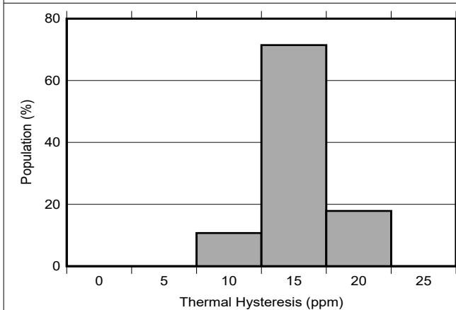
图 6-17. REF54250 热迟滞分布 ( 0^\circ\text{C} 至 70^\circ\text{C} )
