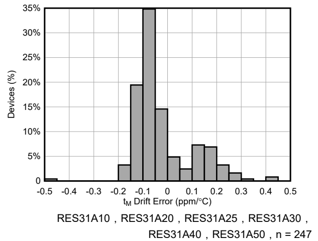
图 5-26. \text{TCR}_M 温度系数分布
