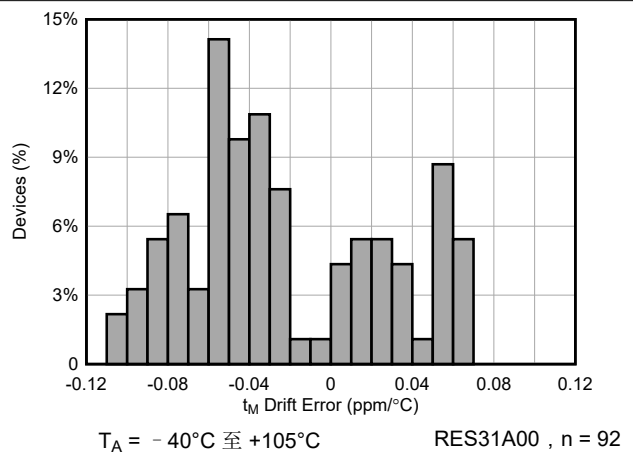
图 5-28. RES31A00 \text{TCR}_M 温度系数分布
