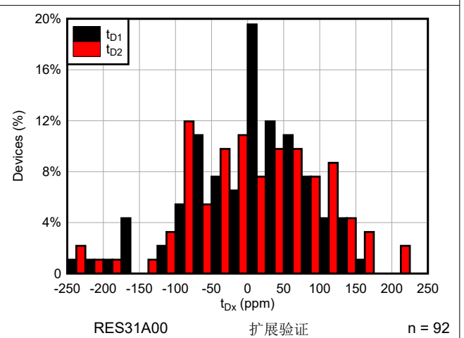
图 5-10. t_{Dx} 分布
