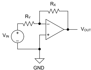
图 8-12. V_{OUT} = -20 \times V_{IN} ，有效电路
