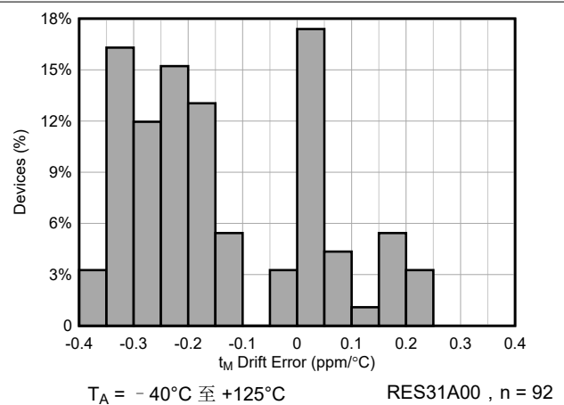
图 5-30. RES31A00 \text{TCR}_M 温度系数分布
