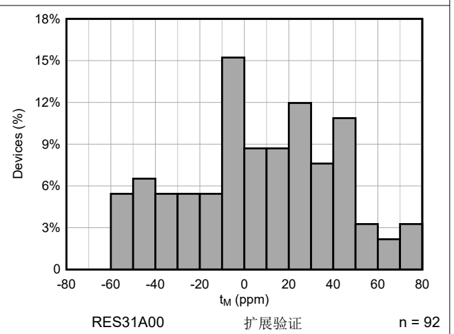
图 5-12. t_M 分布
