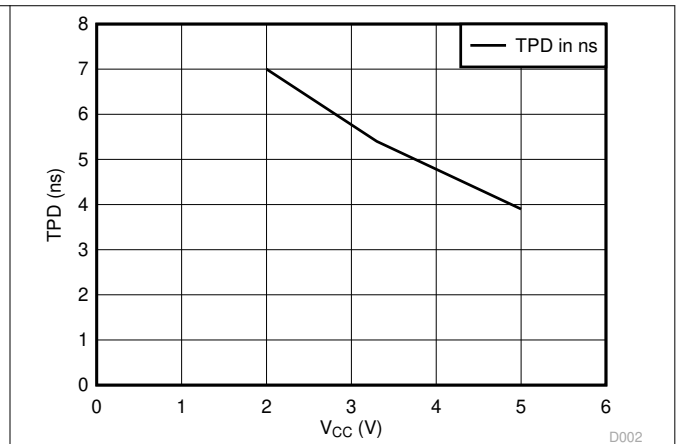
图 5-2. TPD 与 V_{CC} 间的关系
