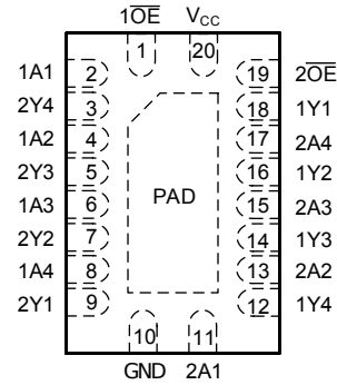
图 4-4. SN74AHC244 RKS 封装；20 引脚 VQFN (顶视图)
