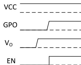
图 7-2. 典型应用时序图
