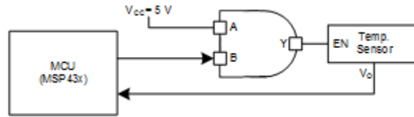
图 7-1. 电源时序应用
