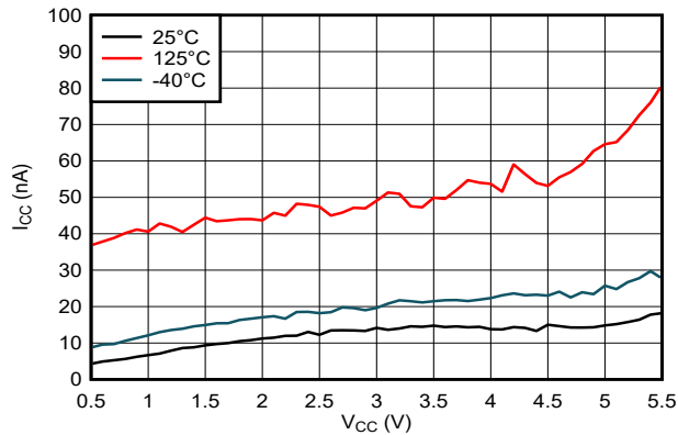
图 6-1. 电源电流与工作电压间的关系
