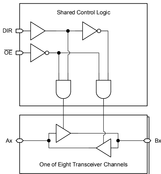
简化逻辑图
