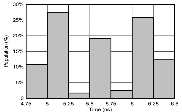
图 6-18. T_{PD} 分布；5V； T_A = -55^\circ\text{C} 至 125^\circ\text{C} (40 个样本)
