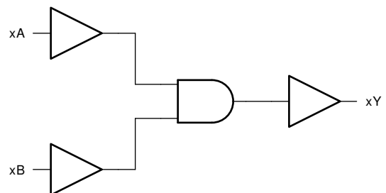
简化逻辑图
