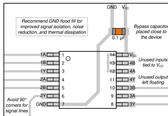
图 9-3. 示例布局 SN54SC4T08-SEP
