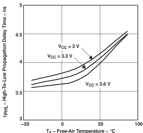
图 5-4. 高电平至低电平传播延迟时间与自然通风温度间的关系
