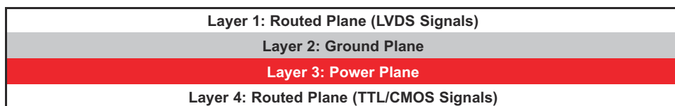
图 10-3. 四层 PCB 板
