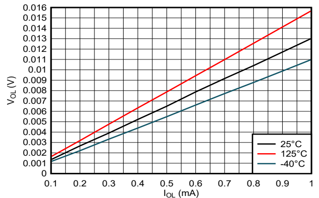
图 5-8. 低电平状态下输出电压与电流间的关系 (1.8V 电源)
