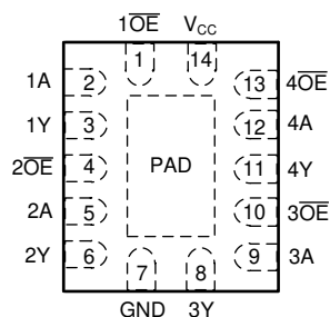
图 4-1. SN74AC126-Q1 BQA 封装 (顶视图)
