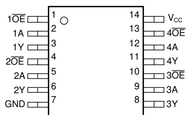
图 4-2. SN74AC126-Q1、PW 封装 (顶视图)
